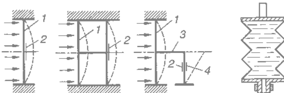
Рис.7.32. Деформационные манометры:
