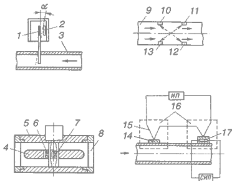
Рис.7.35. Схемы расходомеров:
