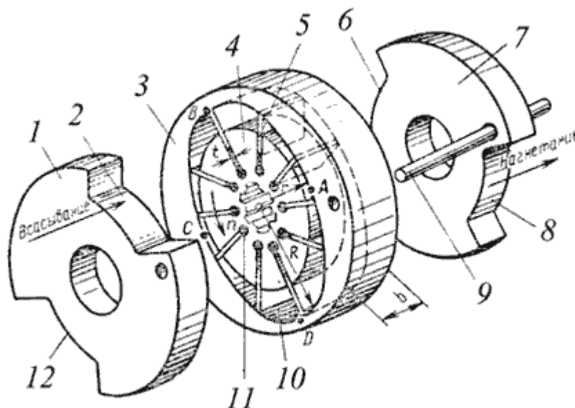
а) 1, 7 - распределительные диски; 3 - статор; 4 - ротор; 5 - пластины; 6, 8 - окна напорной полости; 2, 12 - окна всасывающей полости; 9 - штифт; 10 - внутренняя поверхность статора; 11 - отверстие
