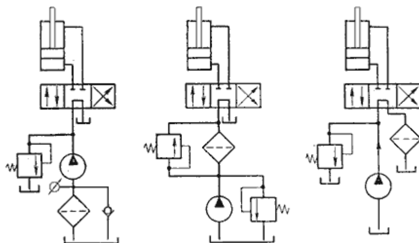
Рис.7.11. Схемы включения фильтров: а - на всасывающей гидролинии; б - в напорной гидролинии; в - в сливной гидролинии
