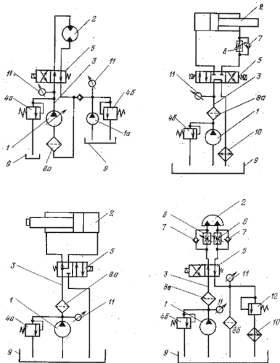
Ри.1.2. Варианты принципиальных схем гидроприводов:
