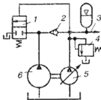
Рис.10.8. Схема системы с двумя спаренными насосами
