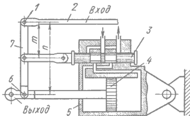
Рис.8.3. Схем гидроусилителя золотникового типа с обратной связью: 1 - шарнир; 2 - тяга; 3 - золотник распределителя; 4 - поршень; 5 - корпус силового цилиндра; 6 - шарнир; 7 - дифференциальный рычаг
