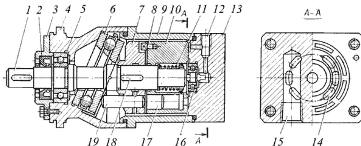
Рис.3.9. Аксиально-поршневой гидромотор типа Г15-2:
