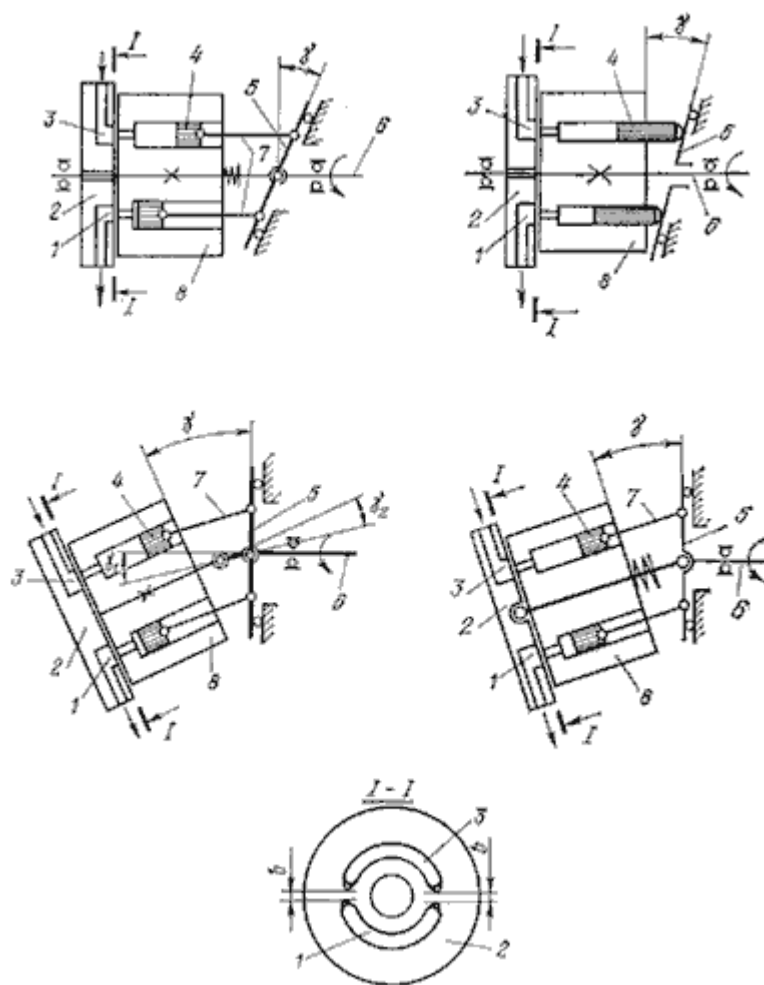
Рис.3.8. Принципиальные схемы аксиально-поршневых насосов:
