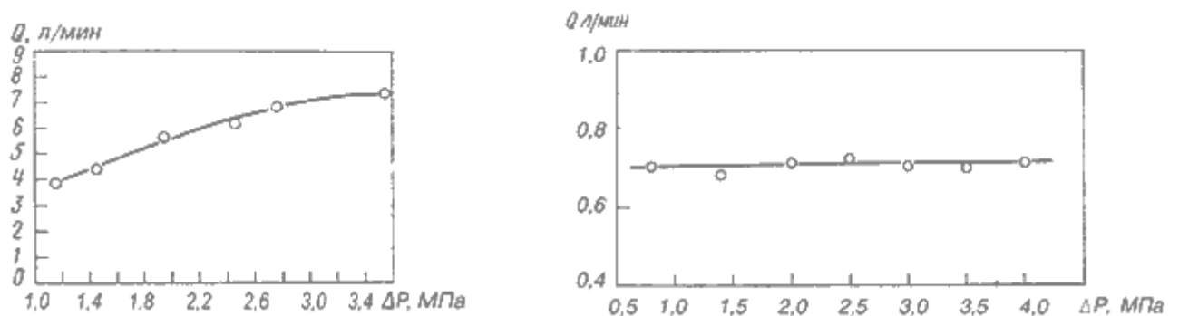
Рис.6.12. Проливочные характеристики а - дросселя Г77-11; б - регулятора расхода Г55-21
