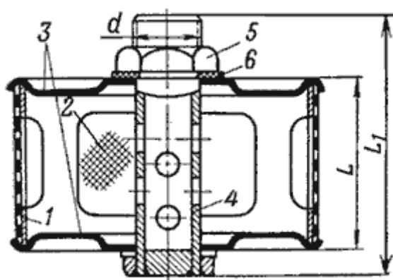
Рис.7.4. Сетчатый фильтр
