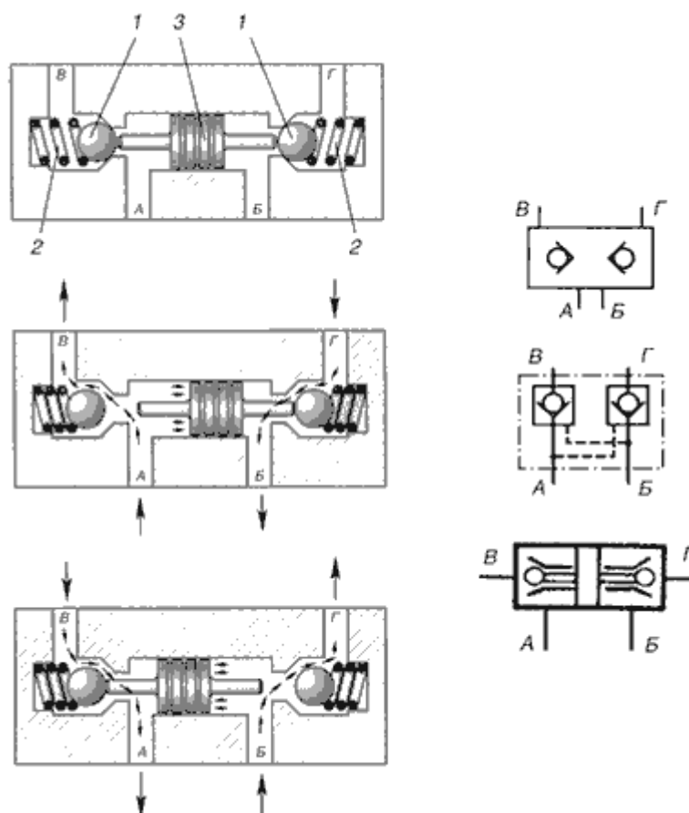
Рис.7.24. Двухсторонний гидрозамок:
