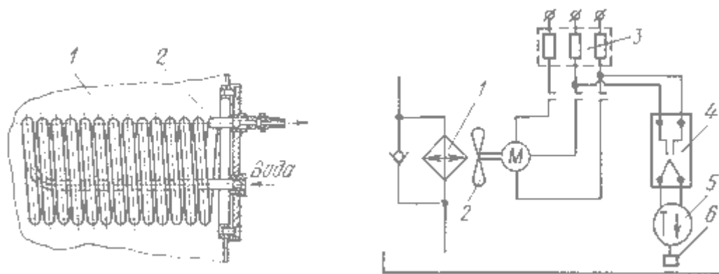
Рис.7.2. Теплообменники:
