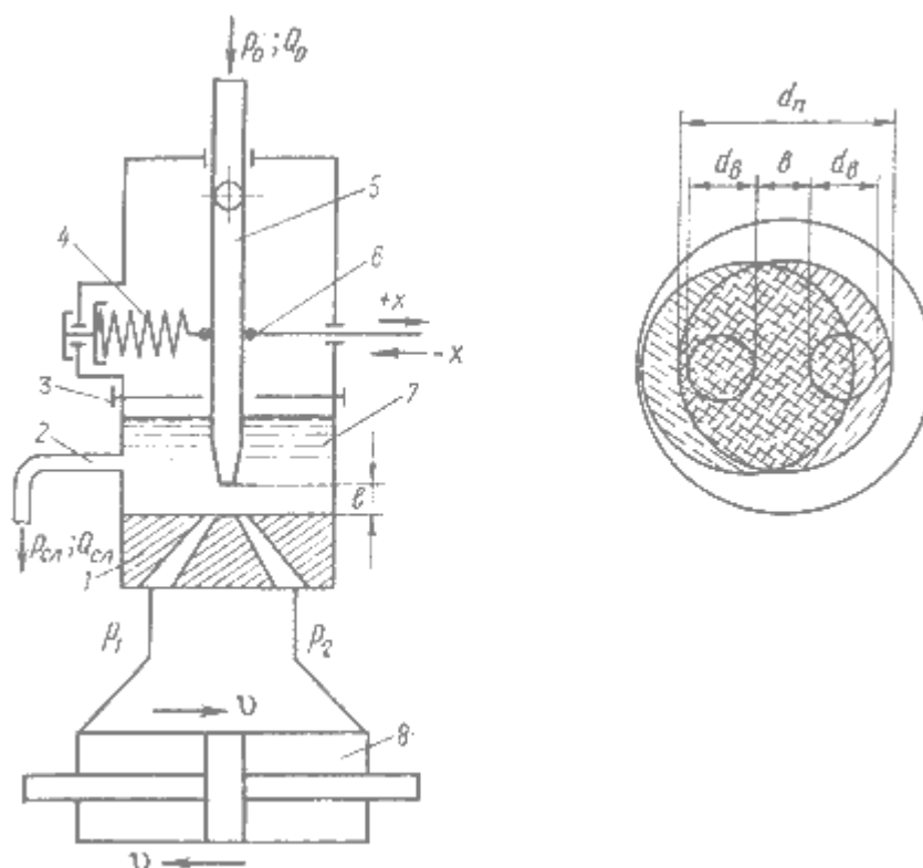
Рис.8.5. Гидроусилитель со струйной трубкой:
