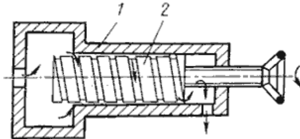
Рис.6.10. Линейный дроссель: 1 - корпус; 2 - винт
