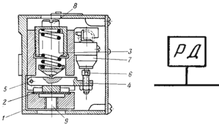
Рис.7.26. Реле давления Г62-2:
