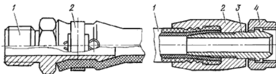
Рис.2.8. Заделка концов рукавов: а - при давлении до 0,5 МПа; б - при давлении свыше 10 МПа 2.5. Расчет гидролиний
