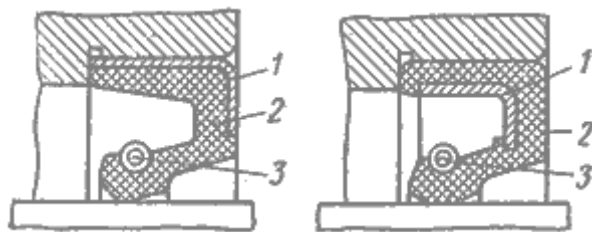
Рис.7.20. Манжеты для уплотнения вращающихся валов: а - с наружным каркасом; б - с внутренним каркасом; 1 - металлический каркас; 2 - манжета; 3 - пружина
