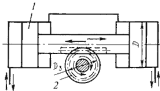
Рис.4.9. Речно-шестеренный механизм
