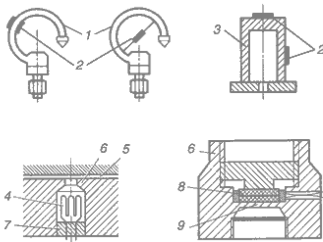
Рис.7.34. Электрические манометры:
