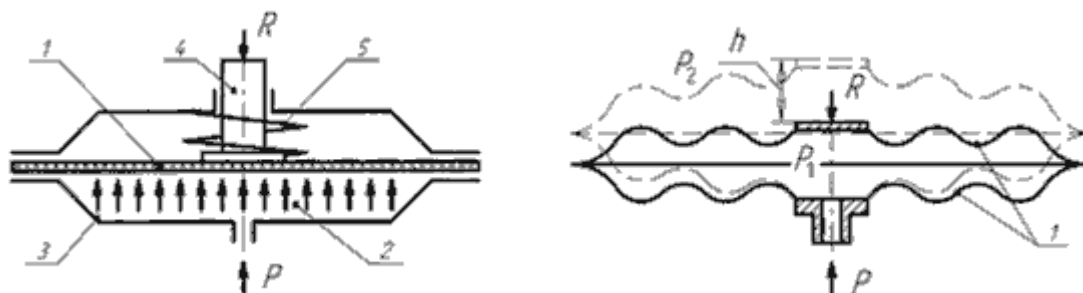
Рис.4.1. Схемы мембран:
