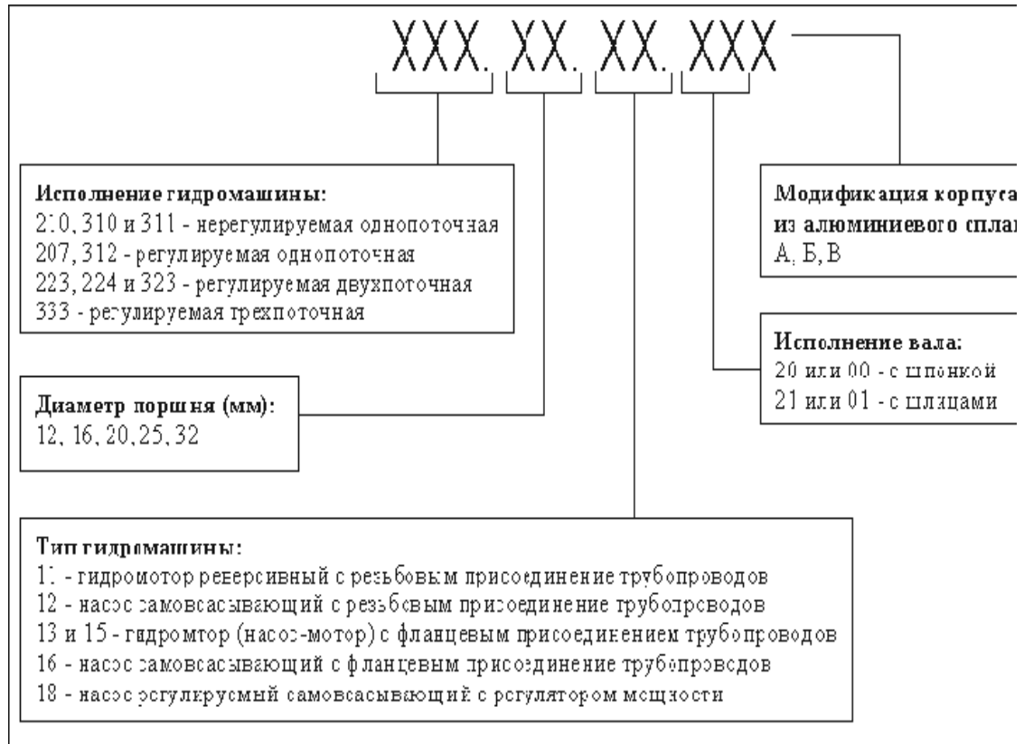
Рис.3.11. Структура условного обозначения аксиально-поршневых гидромашин серий 200 и 300
