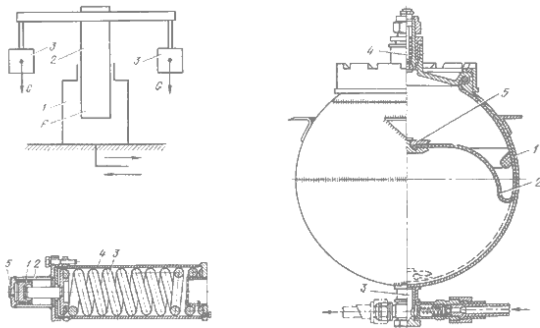
Рис.7.21. Гидроаккумуляторы:
