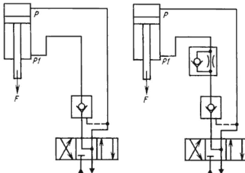
Рис.7.25. Схема установки одностороннего гидрозамка: а - без дросселя с обратным клапаном; б - дросселем и обратным клапаном
