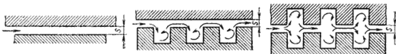
Рис.7.14. Схемы уплотнений: а - щелевого; б, в - лабиринтного
