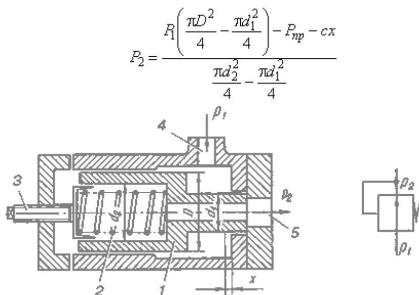
Рис.6.4. Редукционный клапан: а - принципиальная схема; б - условное обозначение
