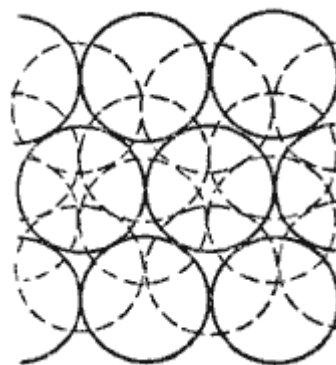
Рис.7.8. Структура фильтроматериала из спеченных шариков
