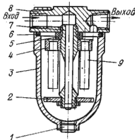
Рис.7.10. Магнитный фильтр типа С43-3:
