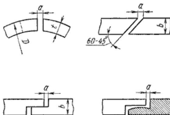
Рис.7.15. Типы стыковых замков металлических колец: а - прямой; б - косой; в, г - ступенчатый
