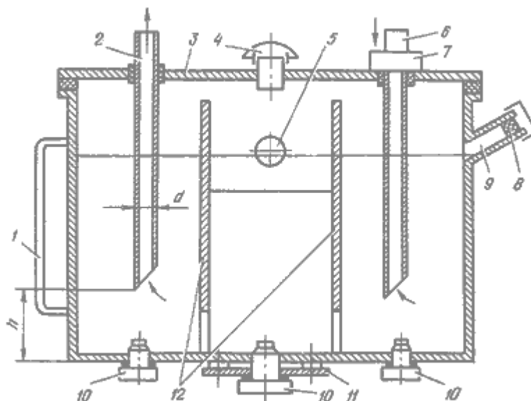
Рис.7.1. Гидробак:
