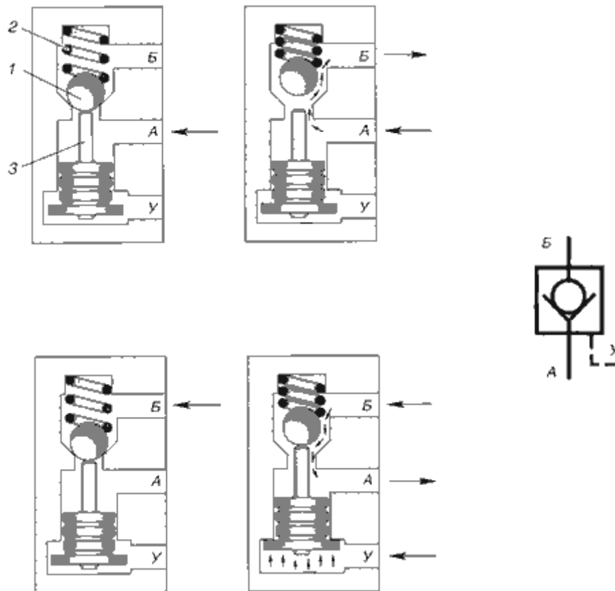
Рис.7.23. Односторонний гидрозамок
