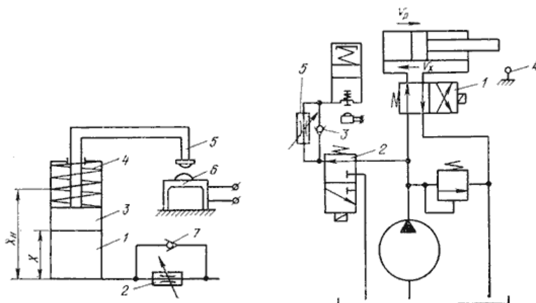
Рис.7.27. Реле времени:
