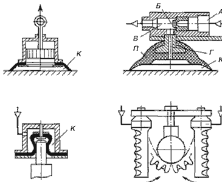
Рис.11.7. Схемы пневмозахватов
