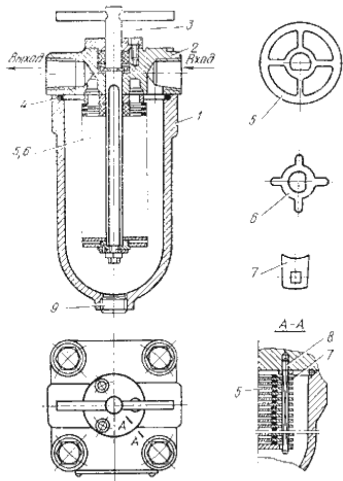
Рис.7.5. Пластинчатый фильтр типа Г41:
