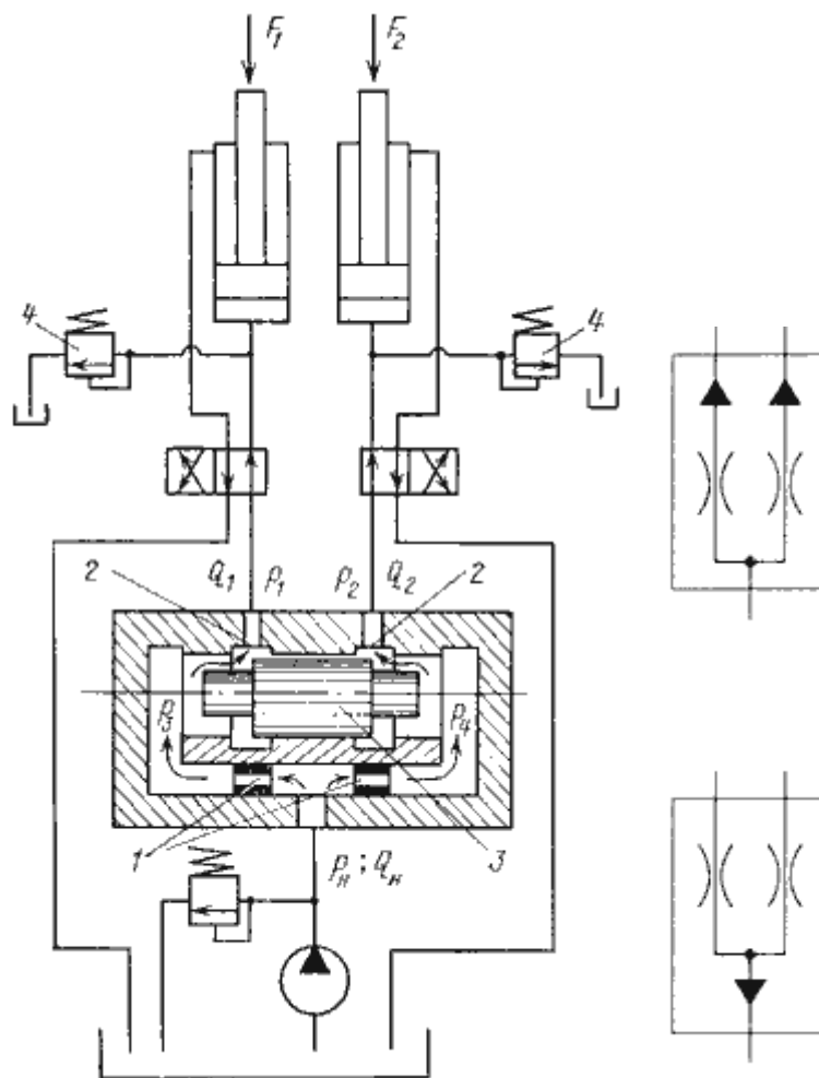
Рис.6.9. Делитель потока: а - принципиальная схема; б - условное обозначение; в - условное обозначение сумматора потока
