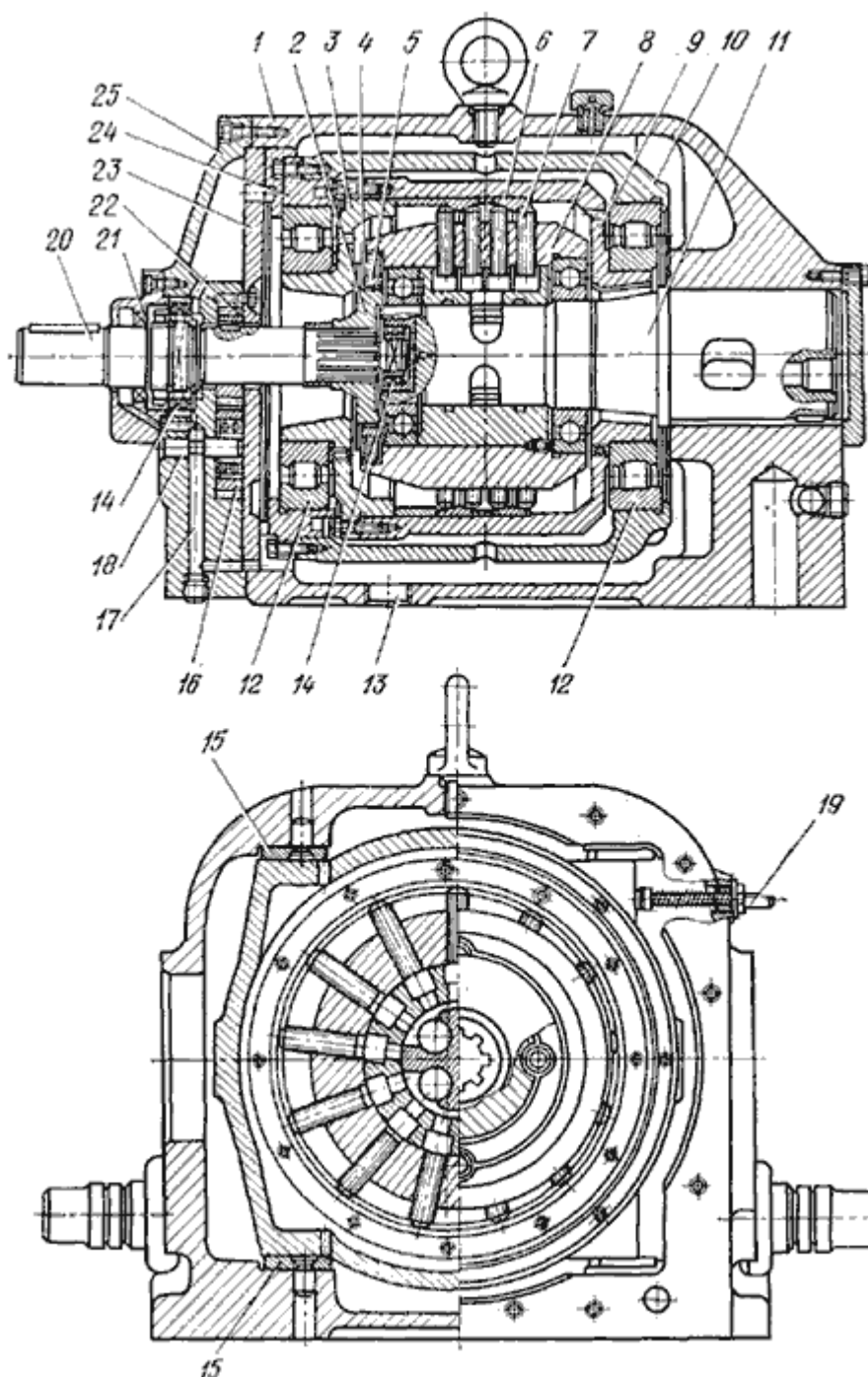
Рис.3.7. Радиально-поршневой насос однократного действия типа НП
