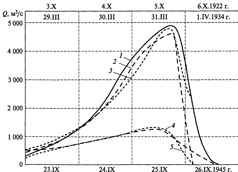
Рис. 6.2. Сравнение рассчитанных (3 и 4) и наблюдаемых гидрографов паводка при прорыве озера Гримсвотн (Исландия) в 1922 (1), 1934 (2) и 1945 гг. (5)
