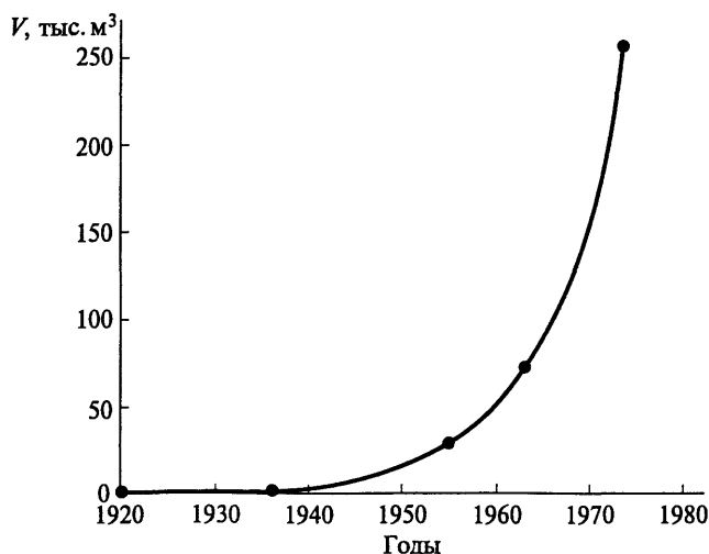
Рис. 6.6. Кривая роста объема моренного озера № 2 у конца ледника Тууксу в бассейне р. Малая Алматинка (Казахстан). Прорыв состоялся 15 июля 1973 г.
