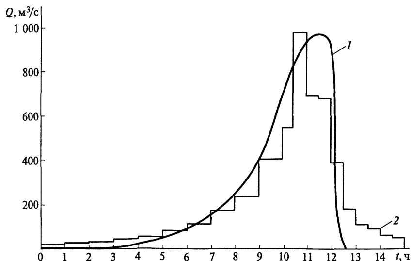
Рис. 6.4. Сравнение рассчитанного (1) и наблюдаемого (2) гидрографов паводка при прорыве озера, подпруженного ледником Медвежийм, 19 июня 1973 г. (бассейн р. Ванч, Памир, Таджикистан)
