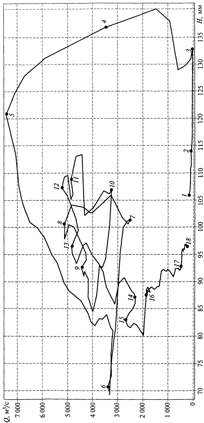
Рис. 3.5. Фазовый портрет состояния бассейна р. Индигирки у села Воронцово ( F = 305 тыс. км 2 ) в 1961 г. На фазовой траектории отмечены номера точек, соответствующих таковым на гидрографе стока (см. рис. 3.6)
