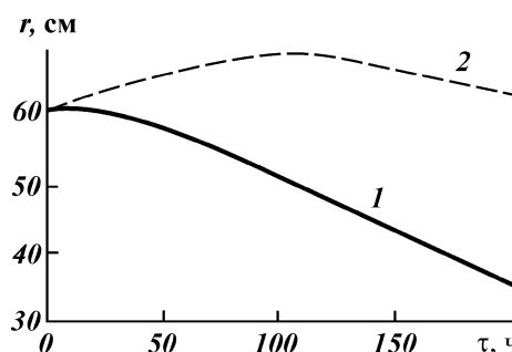
Рис. 6.6. График изменения радиуса r ореола протаивания в породах после прекращения теплового "возмущения"
