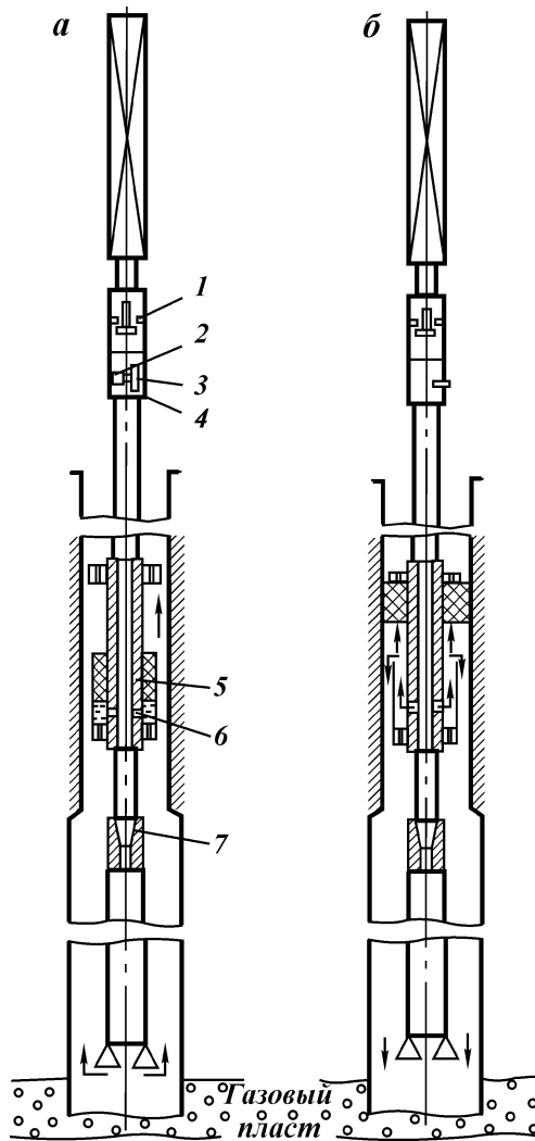
Рис. 8.14. Компонировка бурового инструмента при глушении фонтанов в бурящихся скважинах
