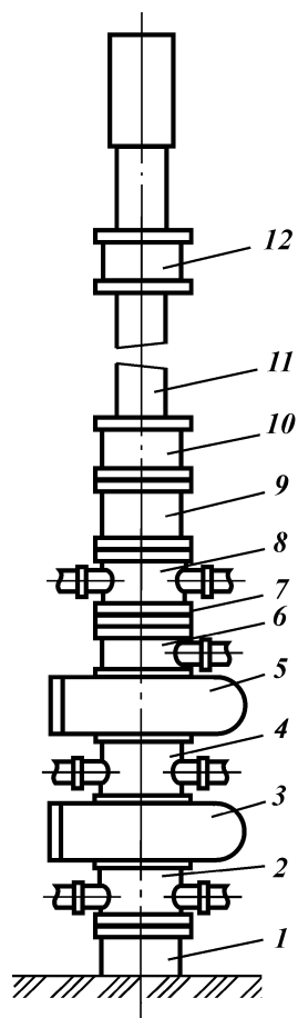
Рис. 8.13. Оборудование устья скважины для спуска буровых труб под давлением: 1 – обсадная колонна; 2, 4, 6, 8 – крестовины; 3, 5 – превенторы; 7 – штуцер; 9 – уплотняющая головка; 10, 12 – шлицевые катушки; 11 – буровая труба
