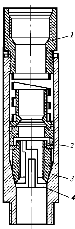
Рис. 9.9. Шлипс с промывкой:
