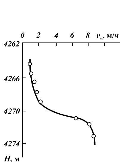
Рис. 4.1. График изменения механической скорости бурения v_m с глубиной z перед выбросом из скважины на Юбилейной площади
