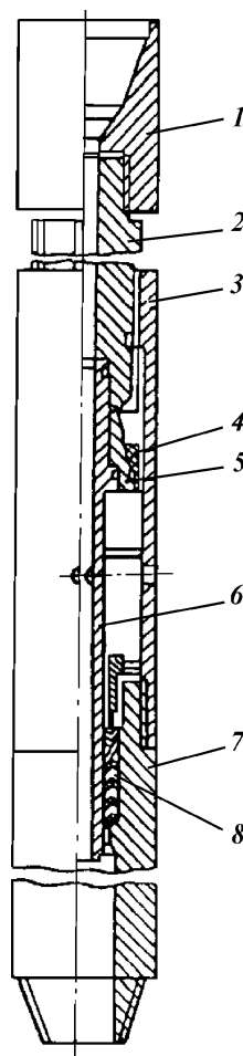
Рис. 7.14. Схема гидравлического ясса открытого типа ЯГ
