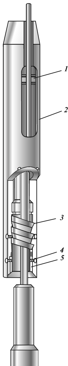
Рис. 9.19. Овершот с боковым окном:
