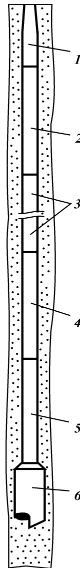
Рис. 9.10. Типичная компоновка ловильной колонны для работы яссами:
