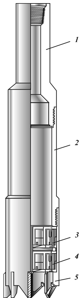
Рис. 9.14. Металлошлакоуловитель колонкового типа
