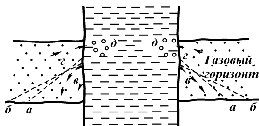
Рис. 4.7. Схема проникновения газа в скважину: а, б – условная зона фильтрата; \cdot – путь фильтрата; \rightarrow – путь газа; \otimes – скопления газа
