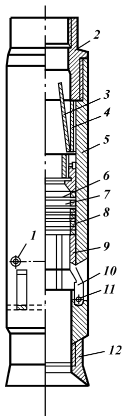
Рис. 9.11. Наружная трубoreзка для бурильных труб
