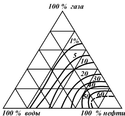
Рис. 2.18. Кривые фазовой проницаемости в тройной системе типа нефть – вода – газ
