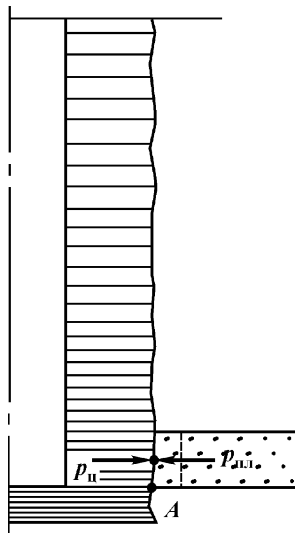
Рис. 4.12. Активное давление цементного раствора p_c на скелет пласта
