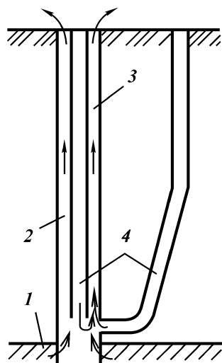
Рис. 8.20. Схема к расчету режимов глушения газовых фонтанов:
