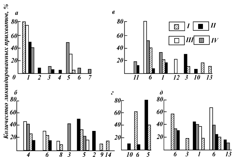
Рис. 7.1. Диаграммы способов ликвидации прихватов.
