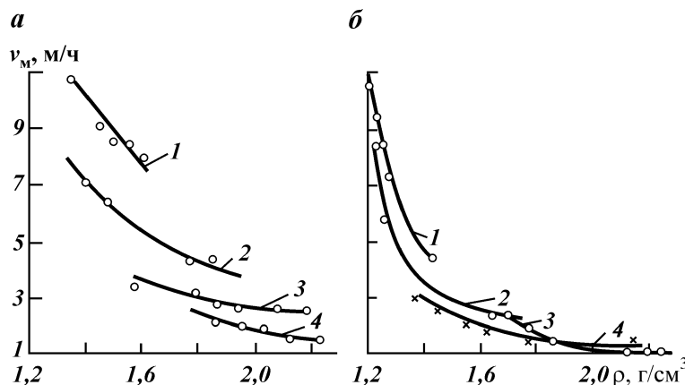
Рис. 10.3. Зависимость механической скорости проходки v_m от плотности \rho бурового раствора: 1 – песчаник; 2 – известняк; 3 – глина; 4 – переслаивание глины и песчаника
