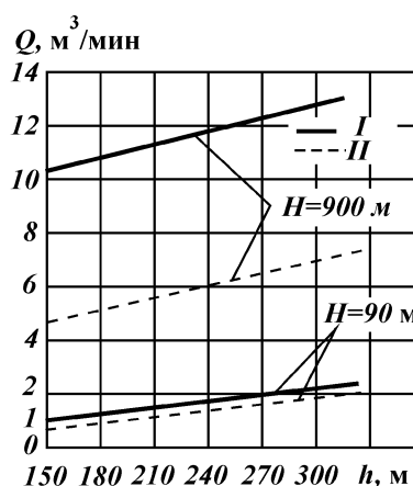
Рис. 4.18. Графики для определения вероятности возникновения выбросов газа при различной глубине моря:
