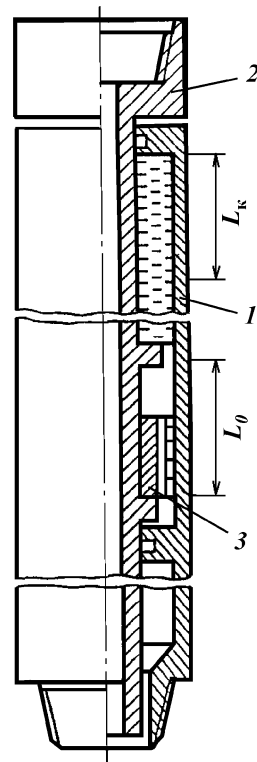
Рис. 7.16. Схема гидравлического ясса конструкции ВНИИБТ: 1 – корпус; 2 – шток; 3 – поршень; L_0 – длина тормозной камеры; L_k – длина свободного хода штока
