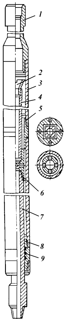
Рис. 7.11. Ясс ударный
