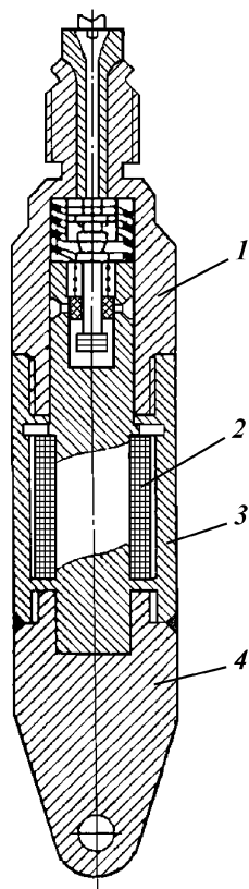
Рис. 7.6. Прихватоопределитель
