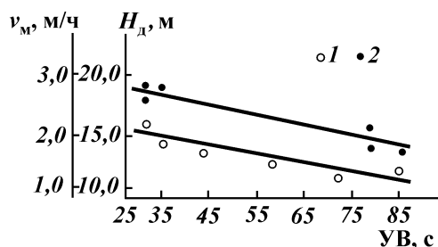
Рис. 10.6. Влияние условной вязкости бурового раствора на скорости проходки v_m и проходки на долото H_d : 1 – проходка H_d ; 2 – скорость v_m
