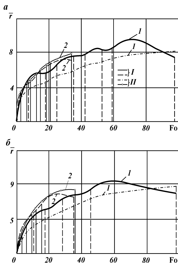
Рис. 6.9. Зависимость безразмерного радиуса \bar{r} ореола протаивания от параметра Fo : a – первый опыт; b – второй опыт; I – эксперимент; II – расчет
