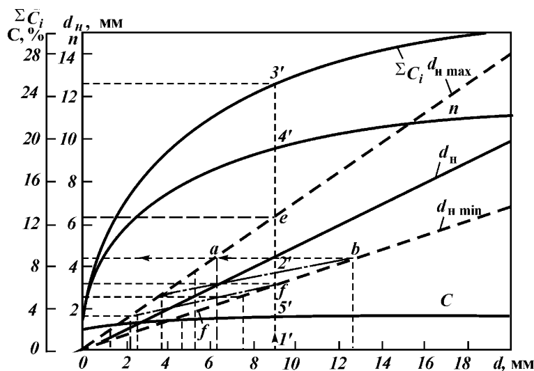
Рис. 2.19. Номограмма для выбора размеров ( d_n , d_{n \max} , d_{n \min} ) концентраций отдельных фракций ( e ) и суммарной концентрации ( \Sigma C_i ), числа фракций ( n ) наполнителей в зависимости от среднего эквивалентного диаметра каналов поглощающего пласта ( d )
