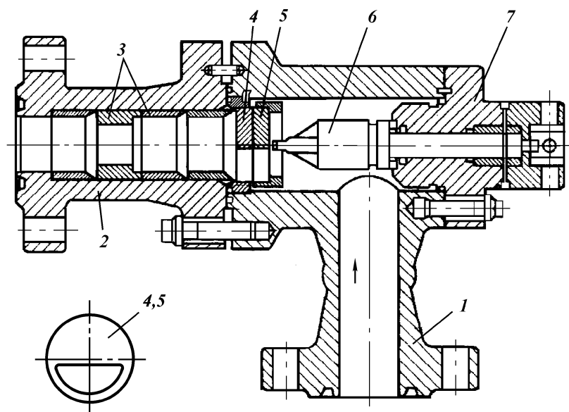
Рис. 10.13. Регулируемый устьевой штуцер фирмы «Свако»: 1, 2 – входной и выходной патрубки; 3 – защитные втулки; 4, 5 – неподвижный и подвижный рабочие диски; 6 – приводной шток; 7 – герметизирующая крышка
