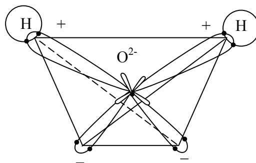
Рис. 2. Схема структуры молекулы воды
