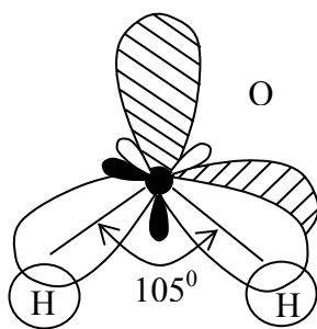
Рис. 2. Схема структуры молекулы воды
