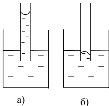
Рис.11. Стеклянная трубка, опущенная в воду (а) и ртуть(б)
