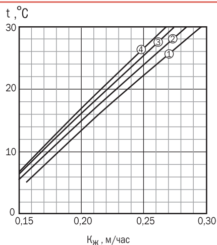
Рис. 1.6. График для определения K_{\text{ж}} при удалении углекислоты в процессе обезжелезивания воды аэрацией. Площадь орошения насадки 90 \text{ м}^3 / (\text{м}^2 \cdot \text{ч}) :
