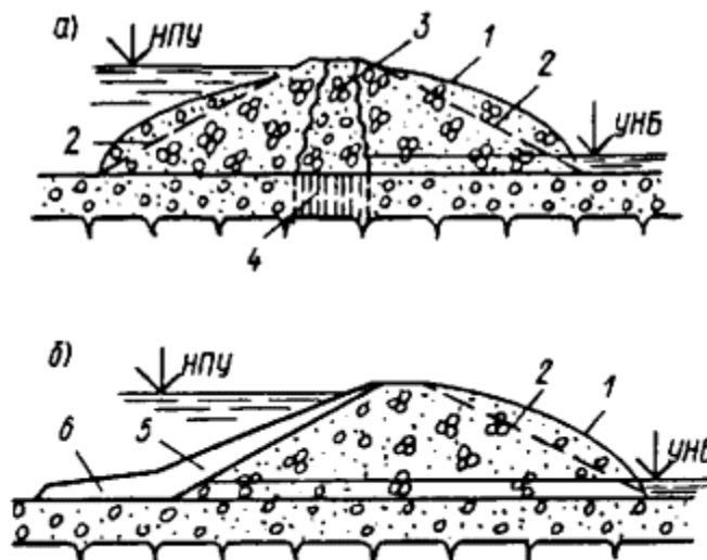
Черт. 7. Виды взрывонабросных плотин
