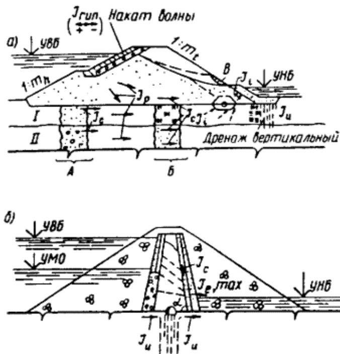
Черт. 9. Фильтрационные деформации в земляных и каменно-земляных плотинах и их основаниях
