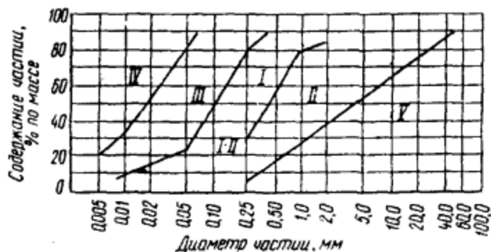
Черт. 5. Группы грунтов, используемых для намыва плотин
