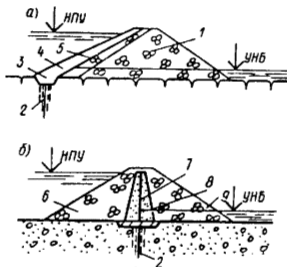
Черт. 8. Виды каменно-набросных плотин
