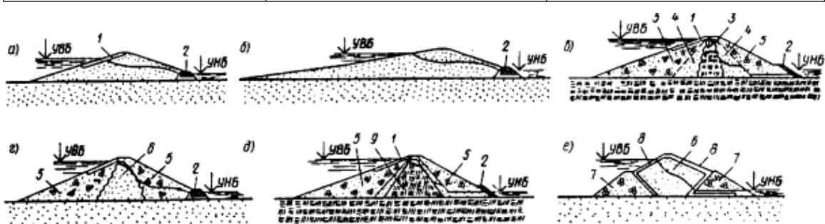
Черт. 3. Виды намывных плотин
