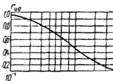
Черт. 3. График зависимости коэффициента порового давления r_{uo} от
