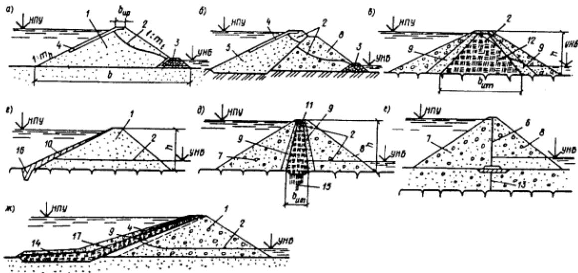
Черт 1. Виды земляных насыпных плотин
