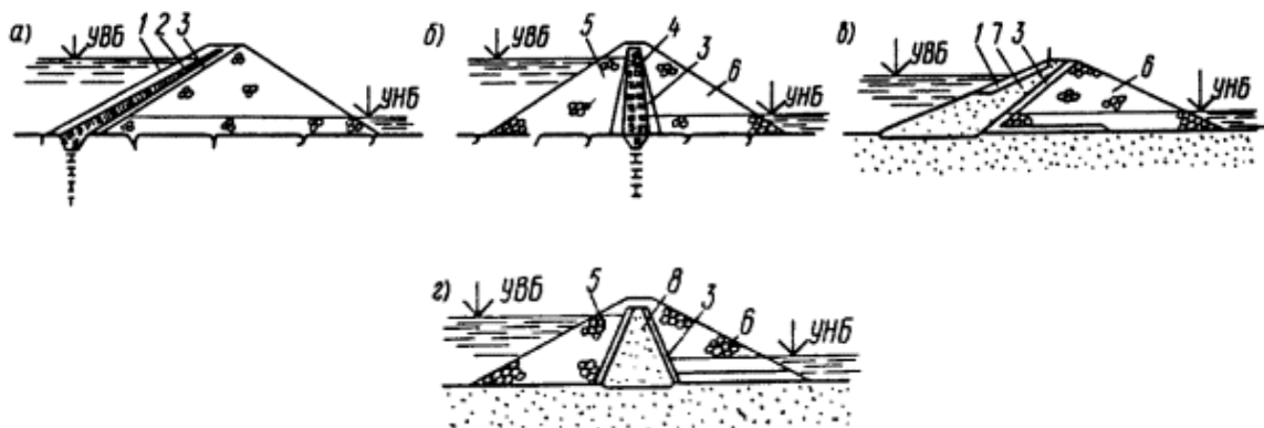
Черт. 6. Виды каменно-земляных плотин
