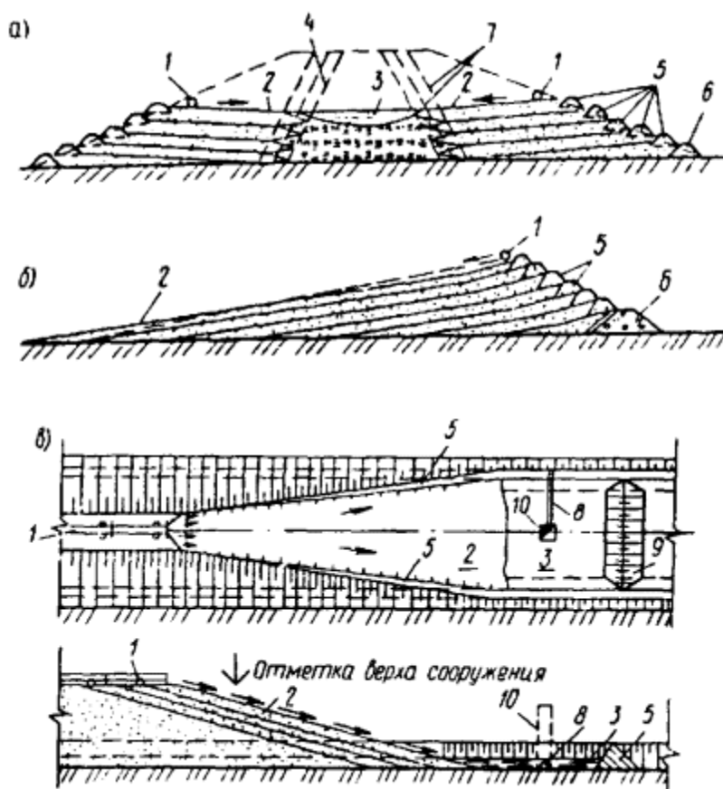
Черт. 4. Основные схемы возведения намывных плотин
