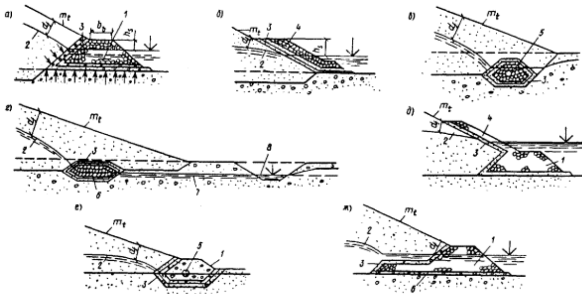
Черт. 2. Схемы основных видов дренажа
