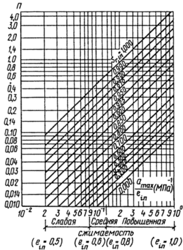
Черт. 2. Номограмма для определения параметра \Pi
