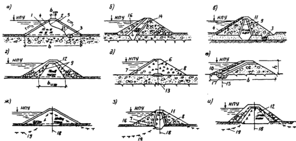
Черт. 1.1. Типы и виды земляных насыпных плотин, возводимых в северной строительно-климатической зоне
