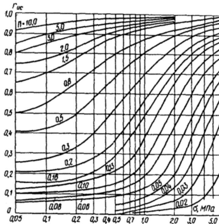
Черт. 1. Номограмма для определения коэффициента парового давления r_{ис}
