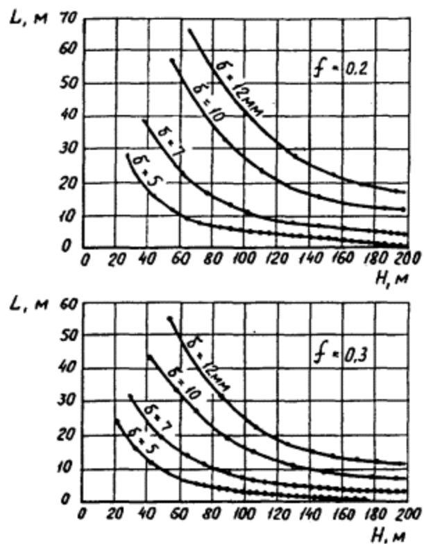
Черт. 1. Зависимость расстояния между горизонтальными швами диафрагмы по высоте L от толщины диафрагмы d , величины коэффициента трения грунта по диафрагме f и высоты диафрагмы H
