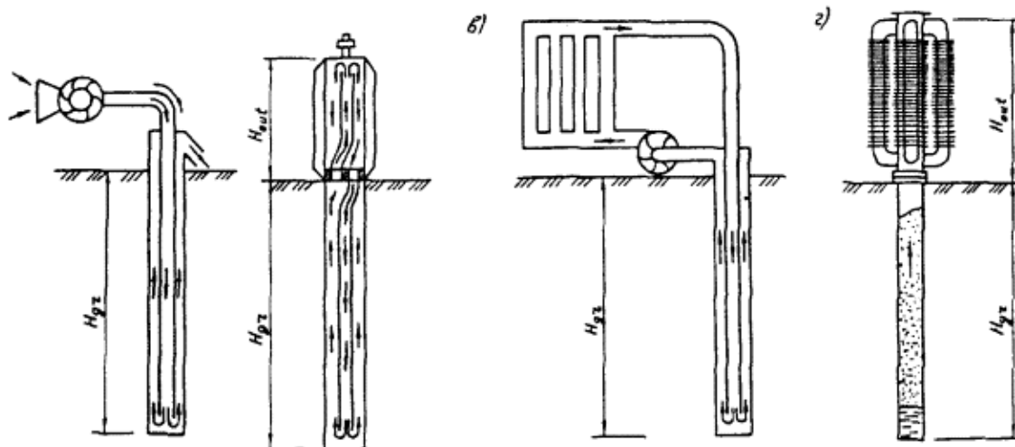
Черт. 2.1. Схемы основных видов СОУ
