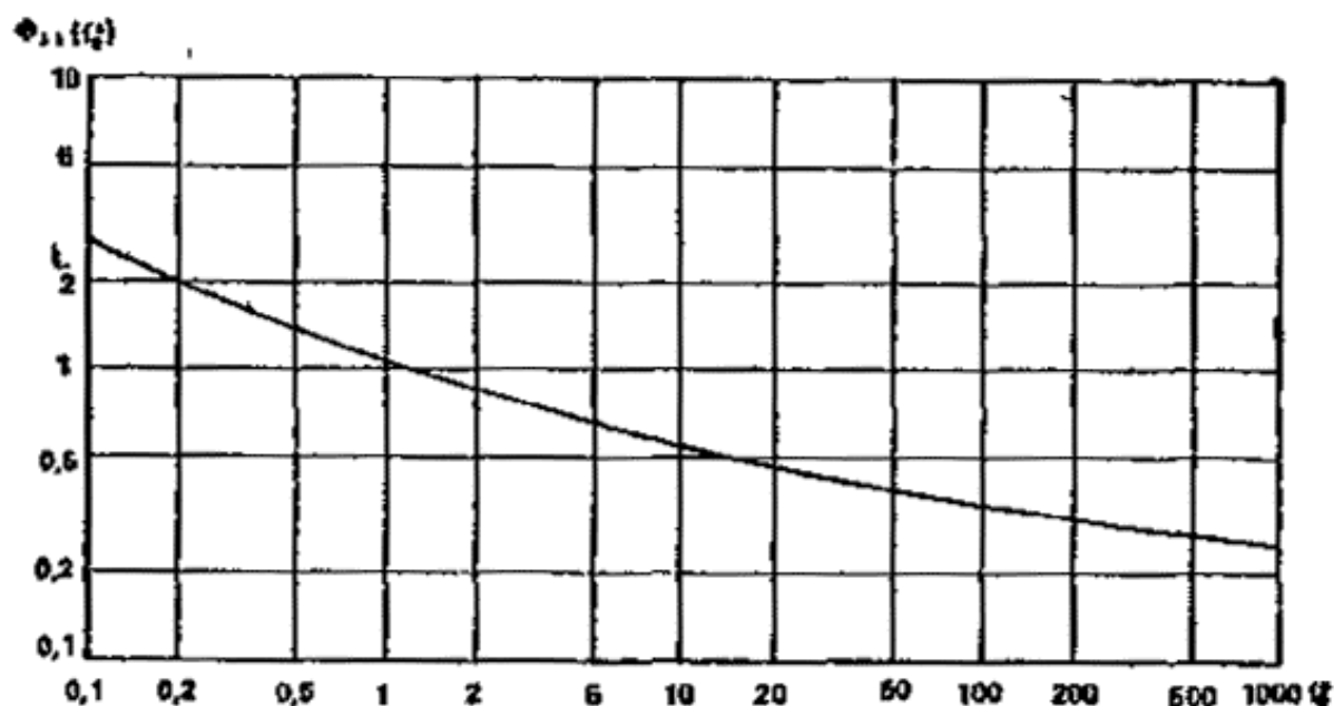
Рис. 88. График функции \Phi_{11}(f_0)
