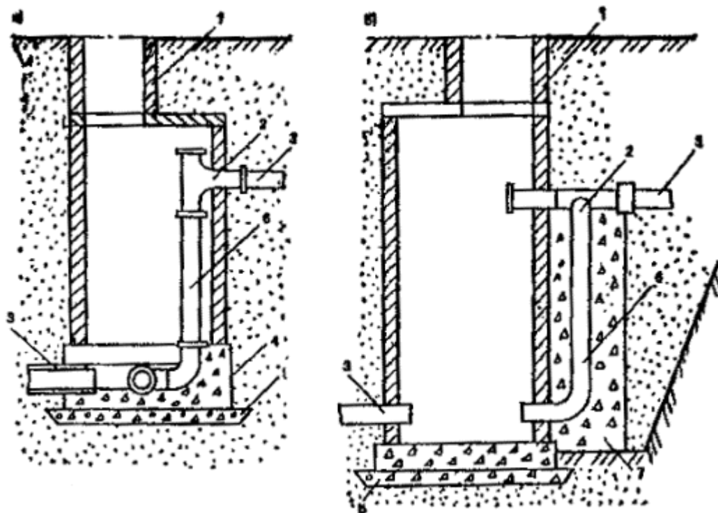
Рис. 61. Конструктивные схемы перепадных колодцев
