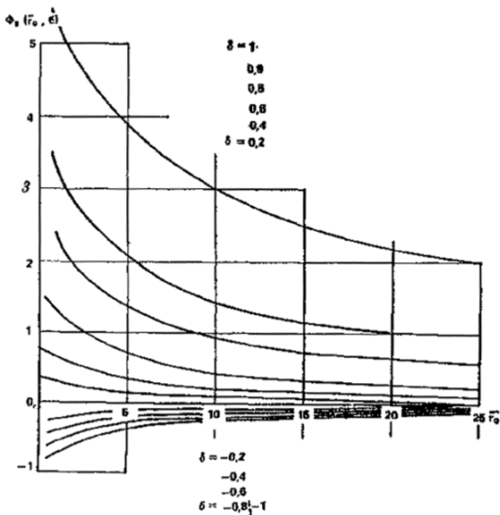
Рис. 85. График функции \Phi_8(\bar{r}_0, \delta)
