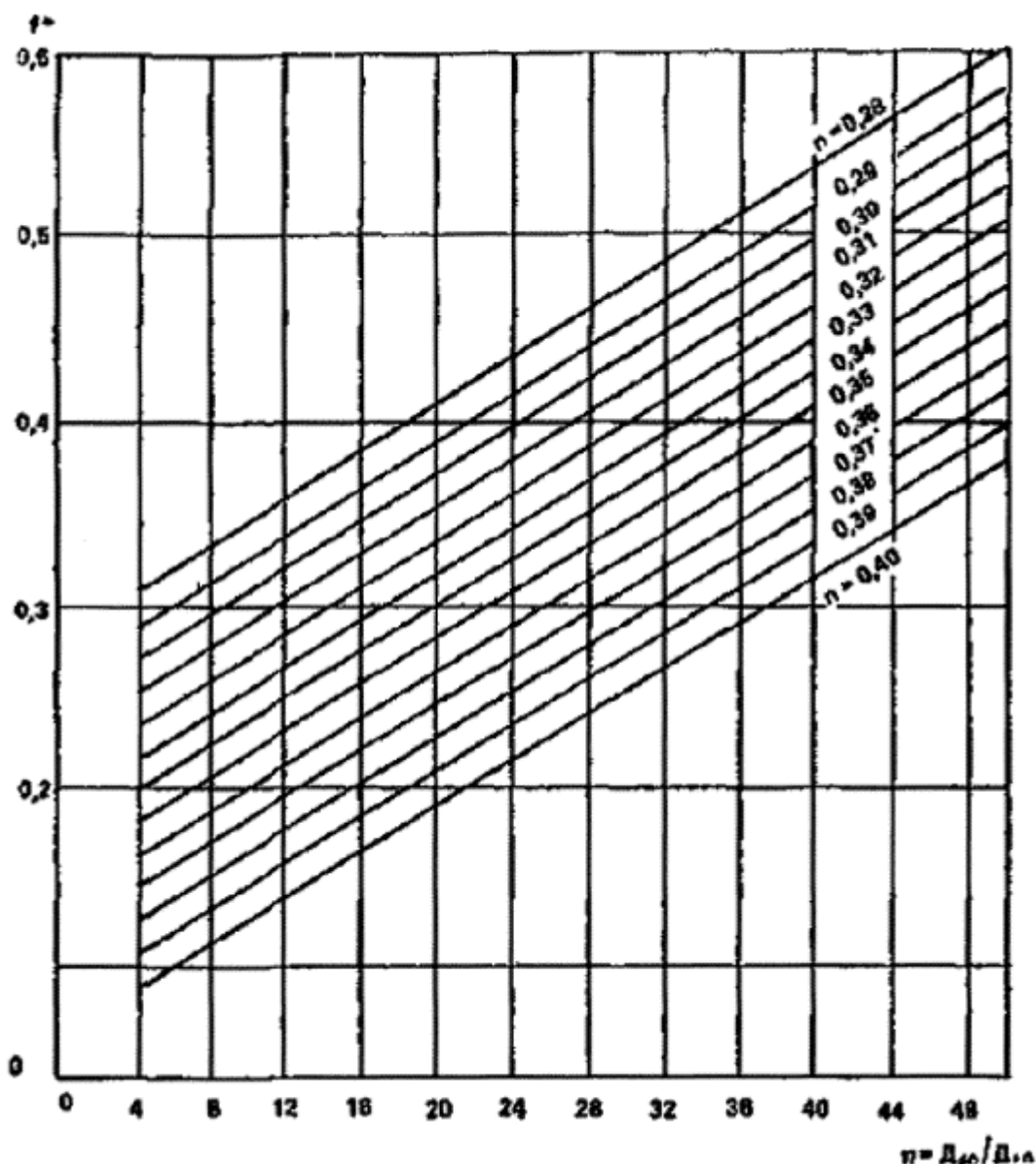
Рис. 127. График f^* = f(\eta)
