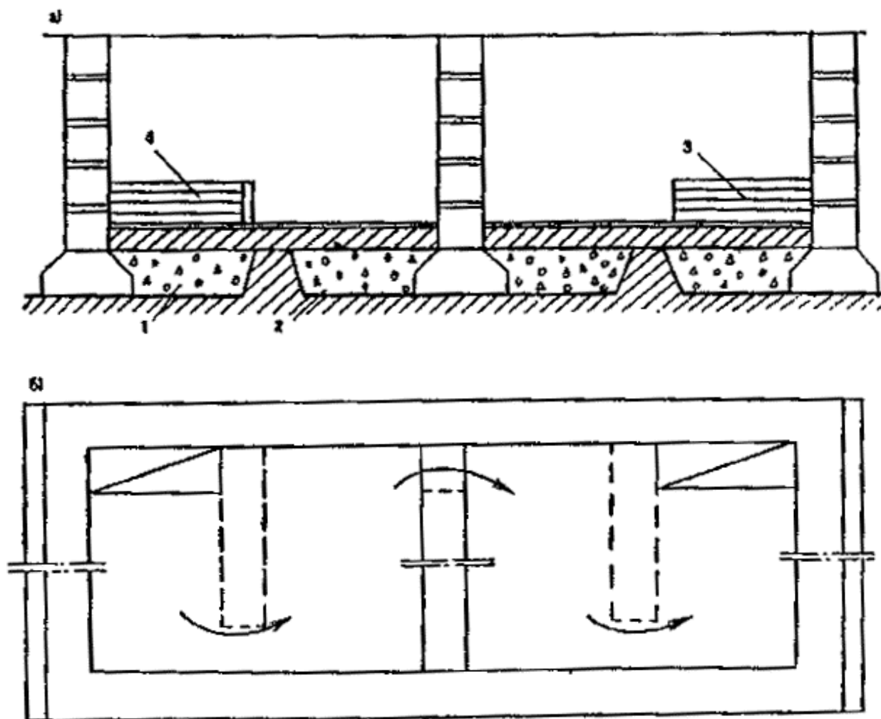
Рис. 30. Пластовый вентиляционный дренаж
