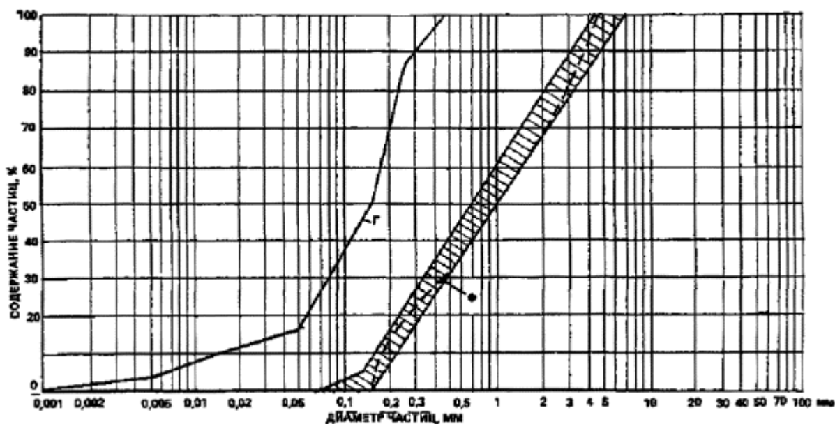
Рис. 136. Кривые гранулометрического состава к примеру подбора зернового состава фильтра для несвязного суффузионного грунта
