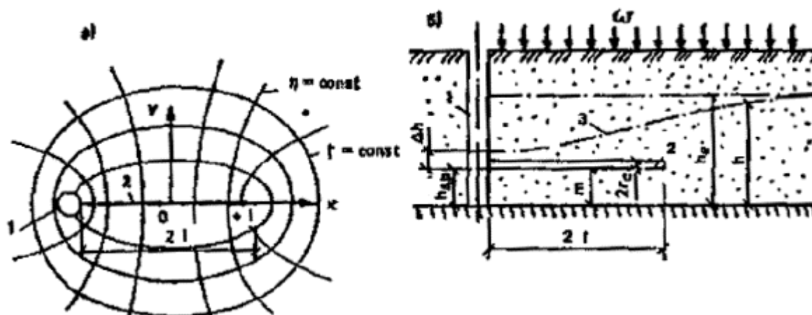
Рис. 94. Схема однолучевого дренажа
