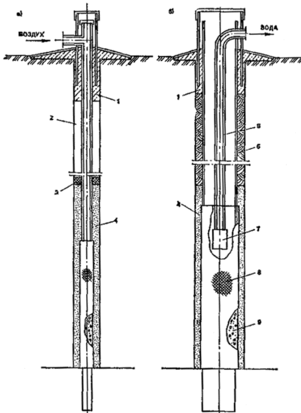
Рис. 55. Скважины пневмонагнетательного дренажа
