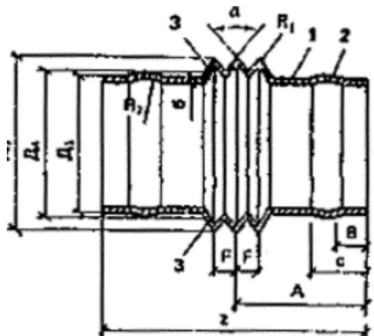
Рис. 40. Конструкция гибкой соединительной муфты
