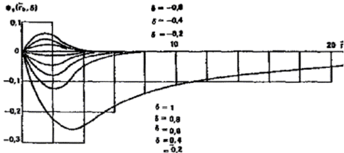
Рис. 86. График функции \Phi_9(\bar{r}_0, \delta)
