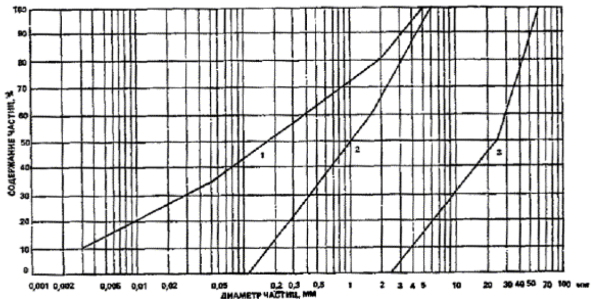
Рис. 137. Кривые гранулометрического состава к примеру подбора зернового состава фильтра для суглинка
