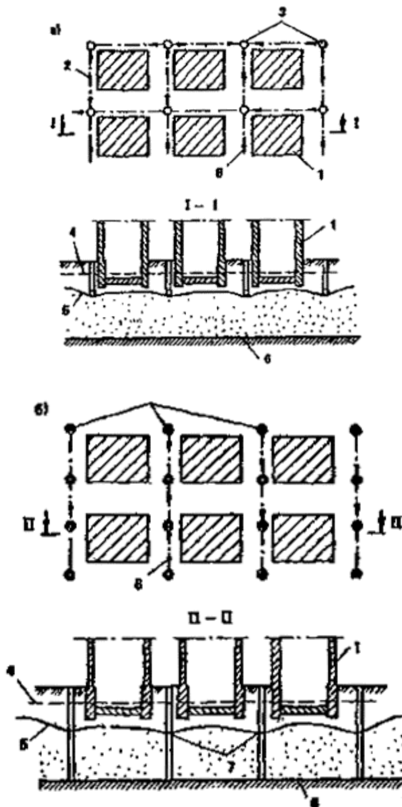
Рис. 58. Схема кольцевого дренажа
