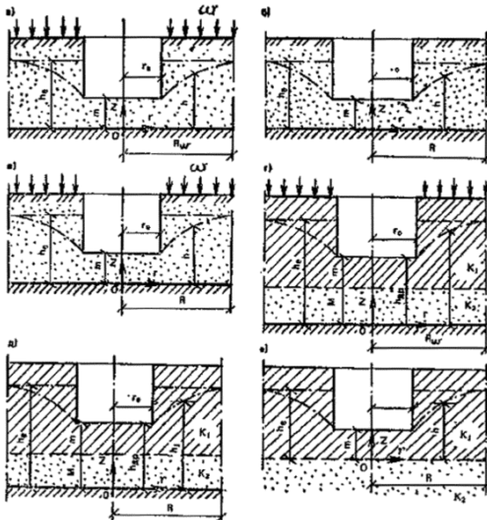
Рис. 90. Схемы пластового дренажа
