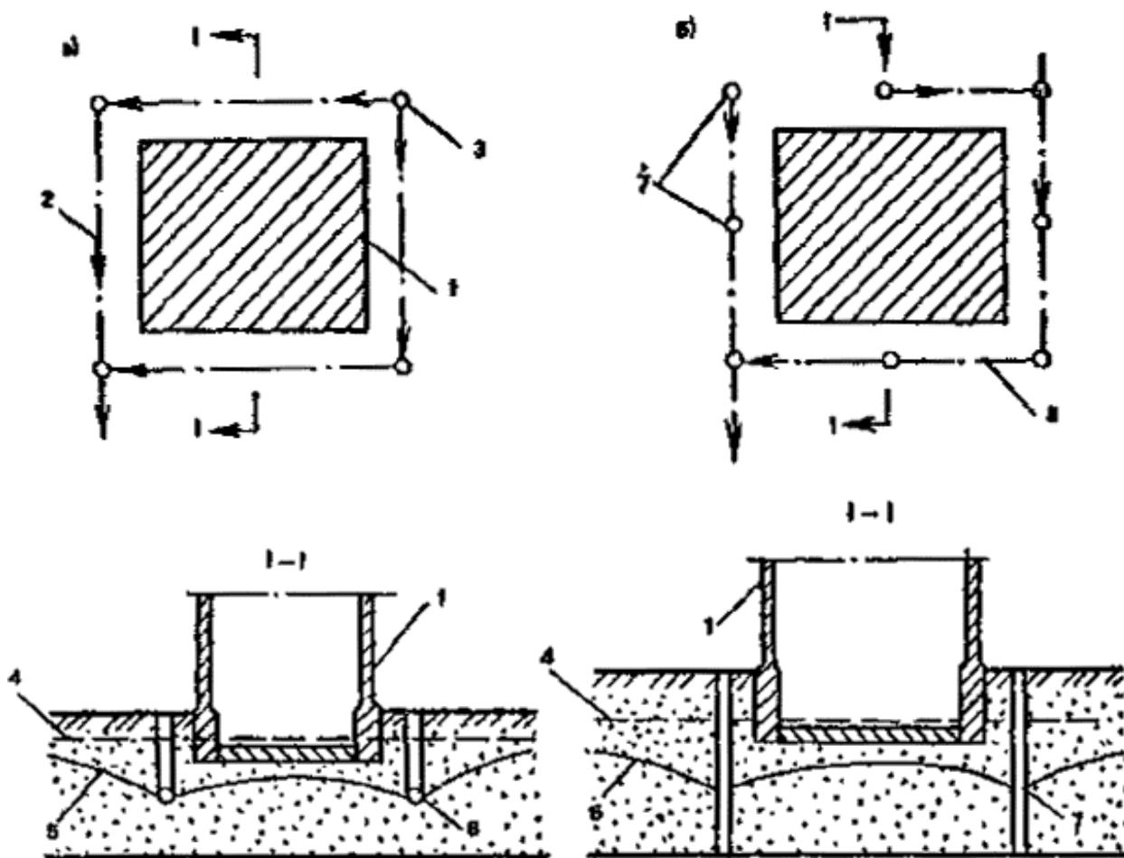
Рис. 59. Схема площадного дренажа
