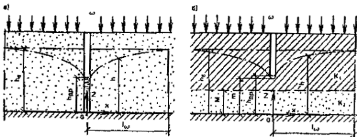
Рис. 72. Расчетные схемы однолинейного дренажа
