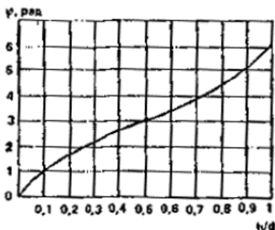
Рис. 123. График зависимости угла \varphi от относительной глубины наполнения трубофильтра водой ( h/d )
