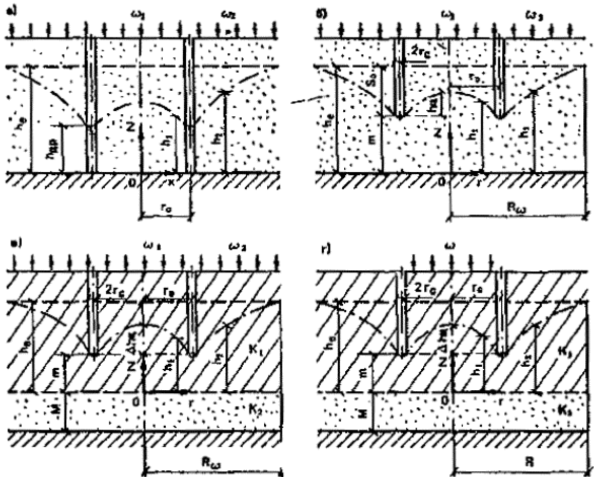
Рис. 77. Схемы кольцевого несовершенного горизонтального дренажа
