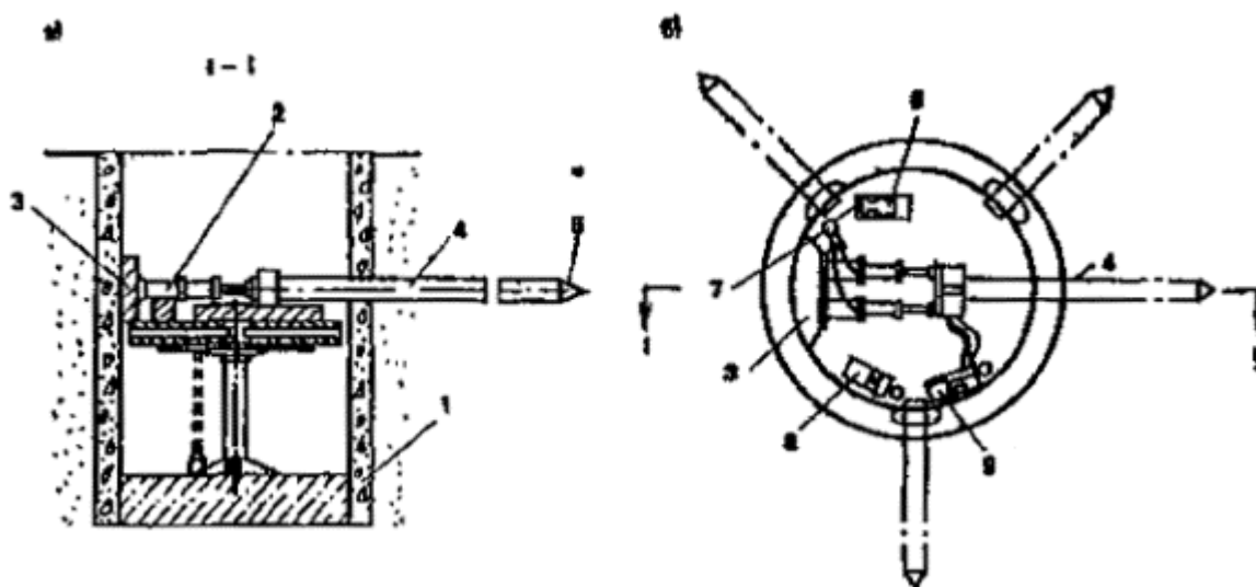
Рис. 44. Схема проходки лучевого дренажа
