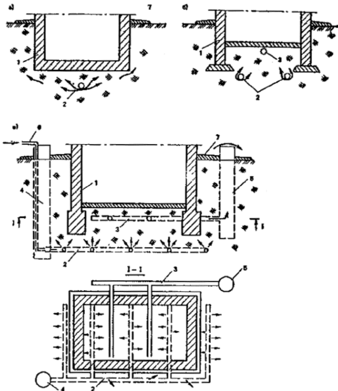
Рис. 54. Конструктивные схемы пневмонагнетательных горизонтальных дренажей
