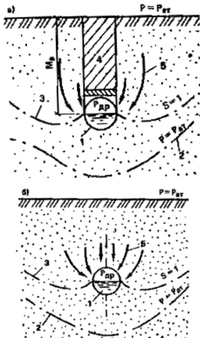
Рис. 103. Схемы к расчету притока воздуха в вакуумный дренаж после его прорыва при наличии (а) и отсутствии (б) защитного экрана
