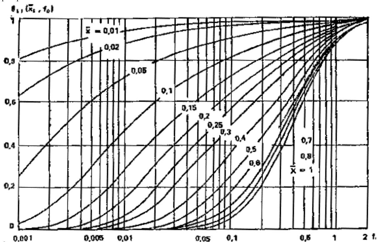
Рис. 102. График функции \theta_{11}(\bar{\xi}, f_0) .
