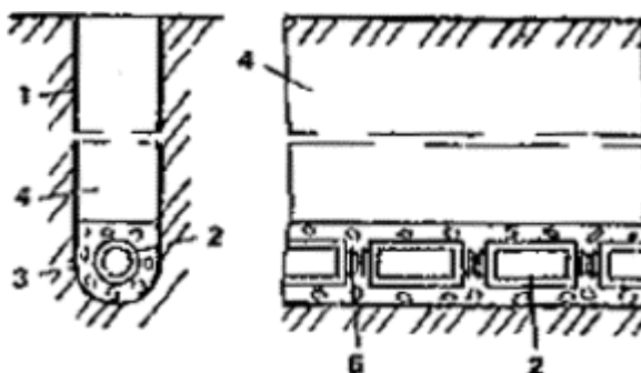
Рис. 41. Конструкция дренажа с применением гибких соединительных муфт
