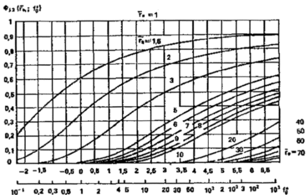
Рис. 89. График функции \Phi_{12}(\bar{r}, f_0)
