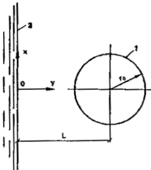
Рис. 84. Схема кольцевого дренажа вблизи прямолинейного контура питания
