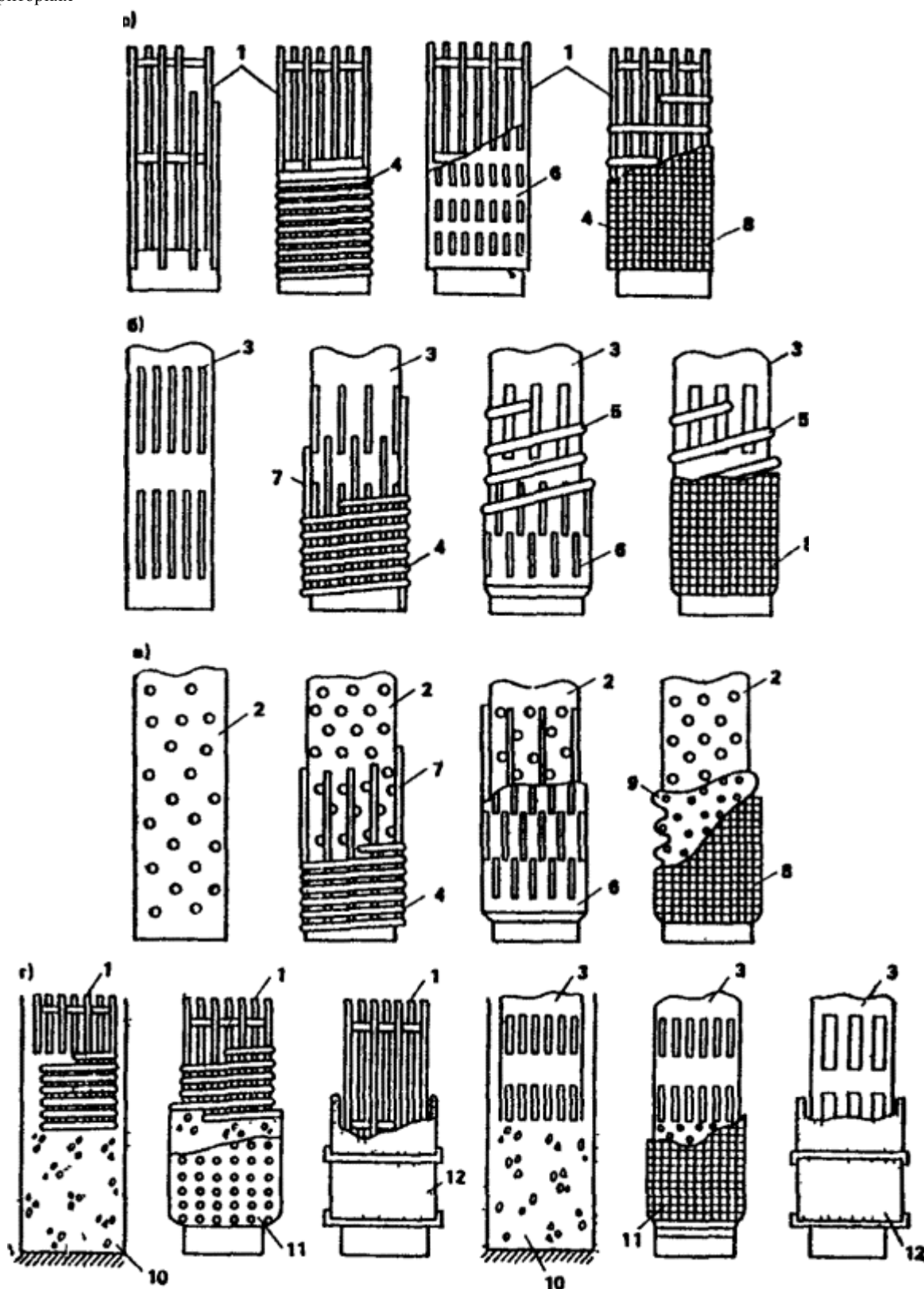
Рис. 48. Конструктивные типы фильтров скважин вертикальных дренажей
