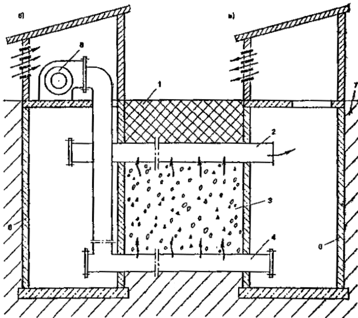
Рис. 31. Конструктивные схемы колодцев вентиляционного дренажа
