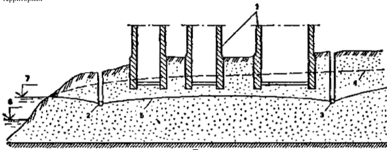
Рис. 57. Схема двухлинейного дренажа
