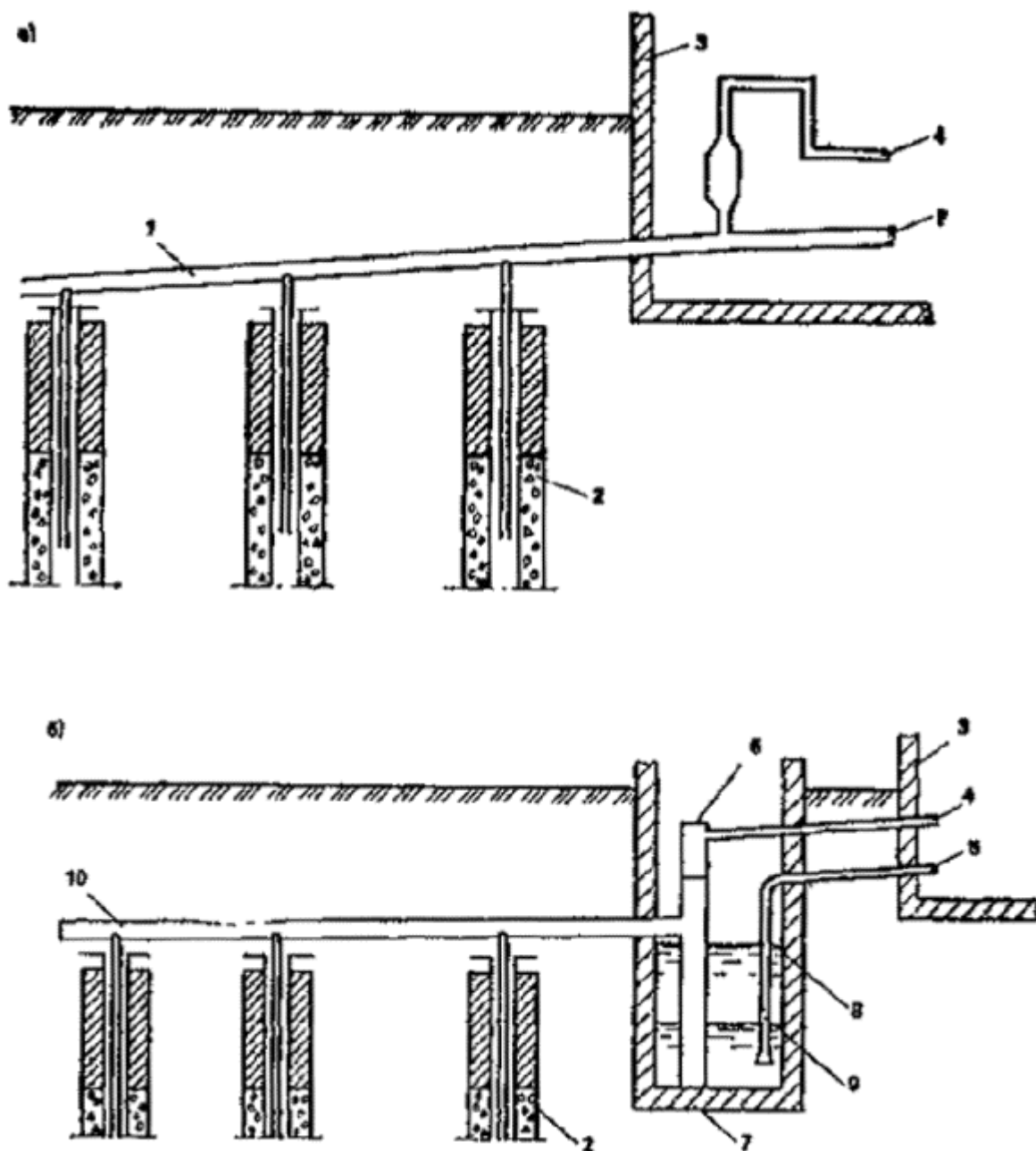
Рис. 52. Схема вертикального дренажа с вакуумным водоподъемом
