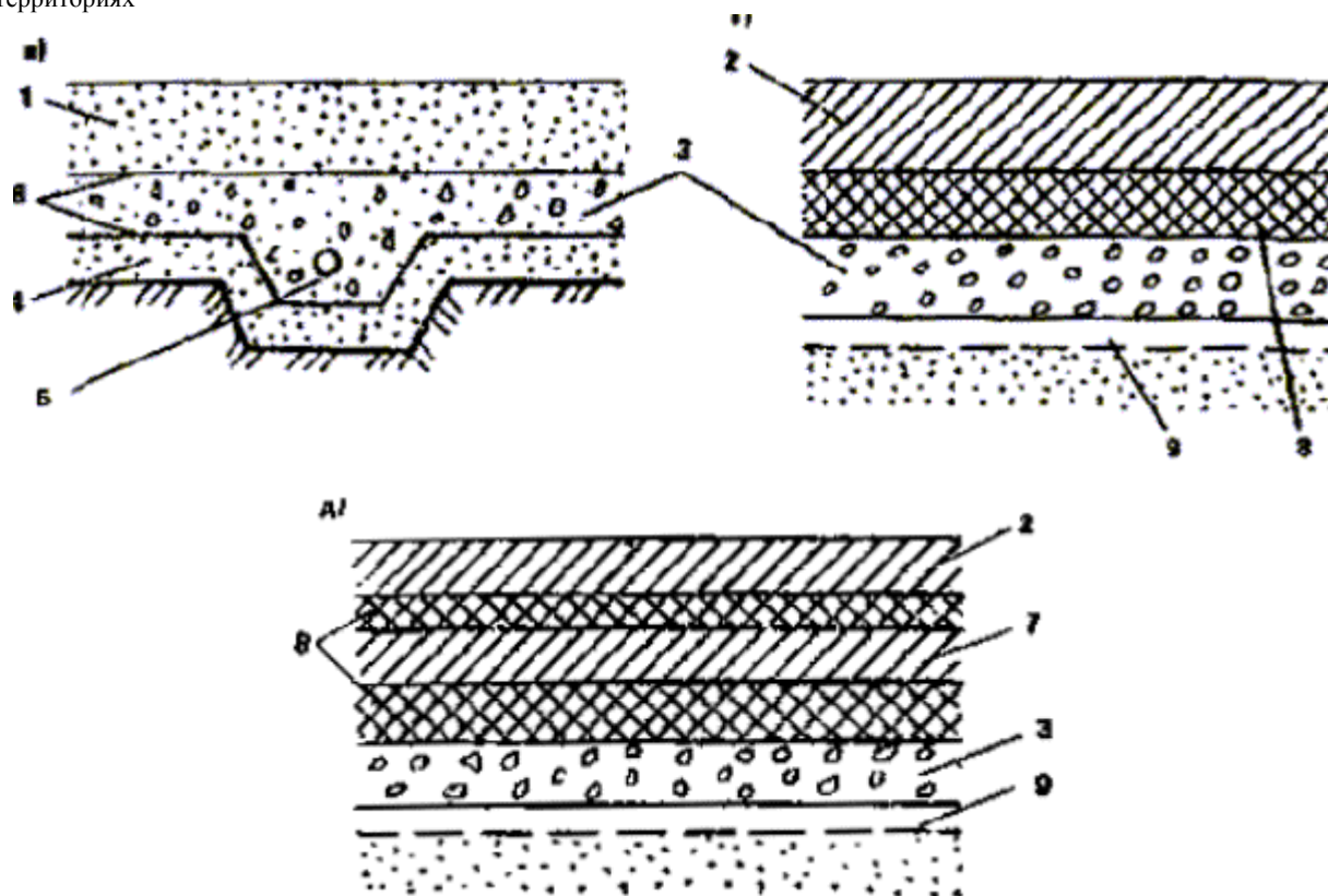
Рис. 34. Схемы противофильтрационных экранов
