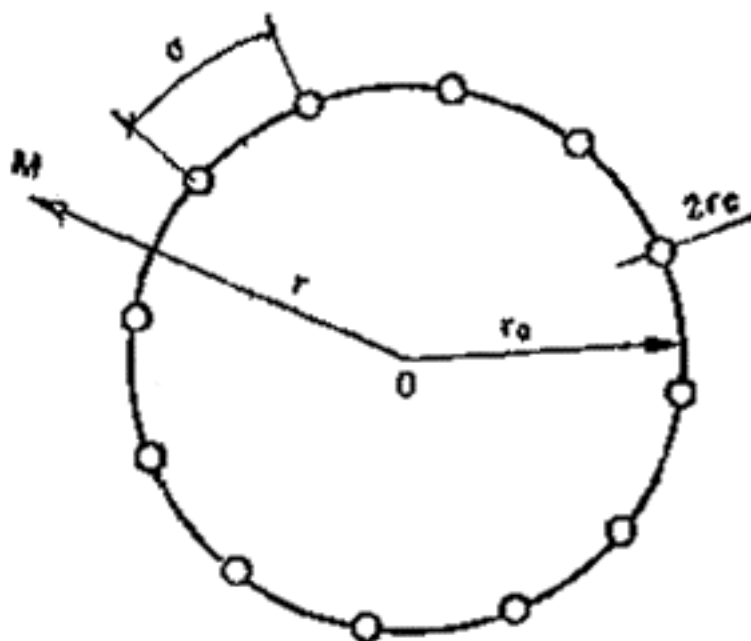
Рис. 115. Кольцевая система скважин в неограниченном пласте
