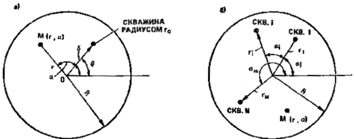
Рис. 106. Одиночная скважина (а) и группа их (б) в водоносном пласте с круговым контуром питания
