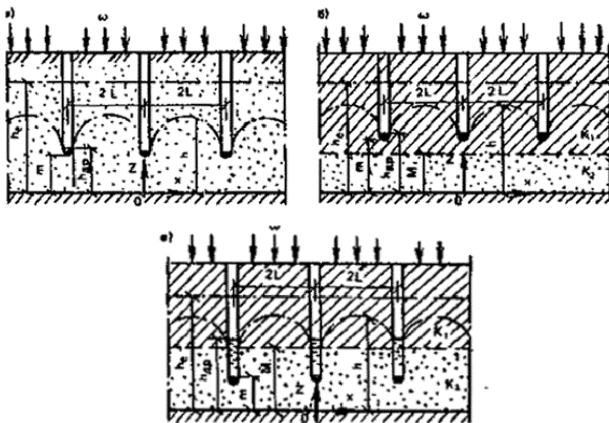
Рис. 70. Схема несовершенного систематического дренажа
