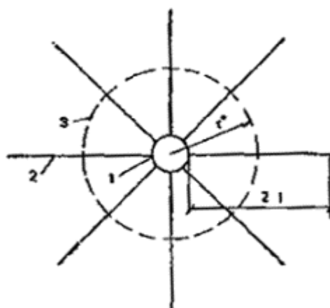
Рис. 95. Схема (в плане) многлучевого дренажа с симметричным расположением дрен-лучей
