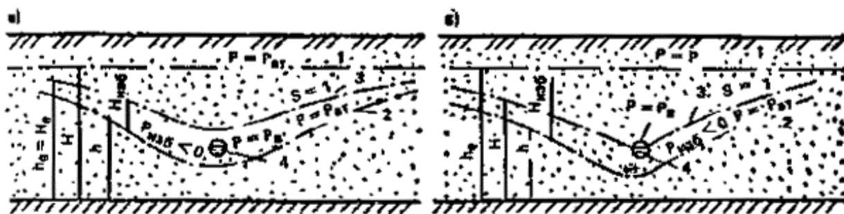
Рис. 99. Схемы к расчету фильтрации к горизонтальной дрине при вакуумировании на первом (а) и втором (б) этапах
