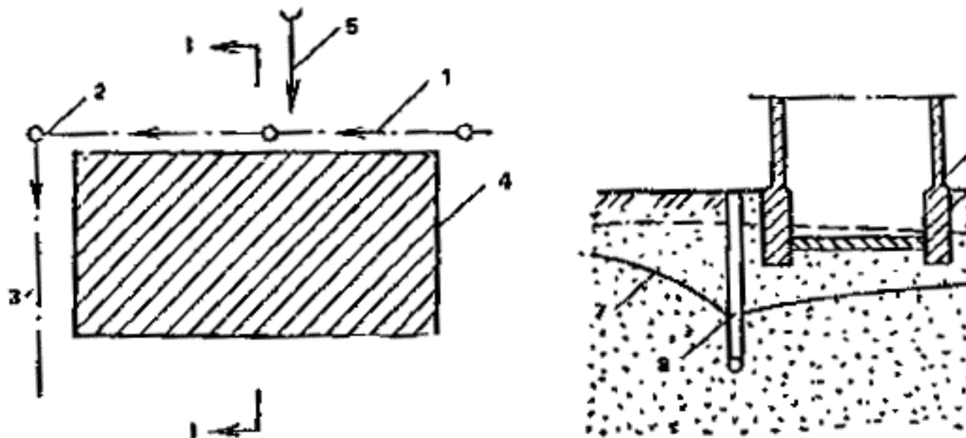
Рис. 35. Схема головного дренажа
