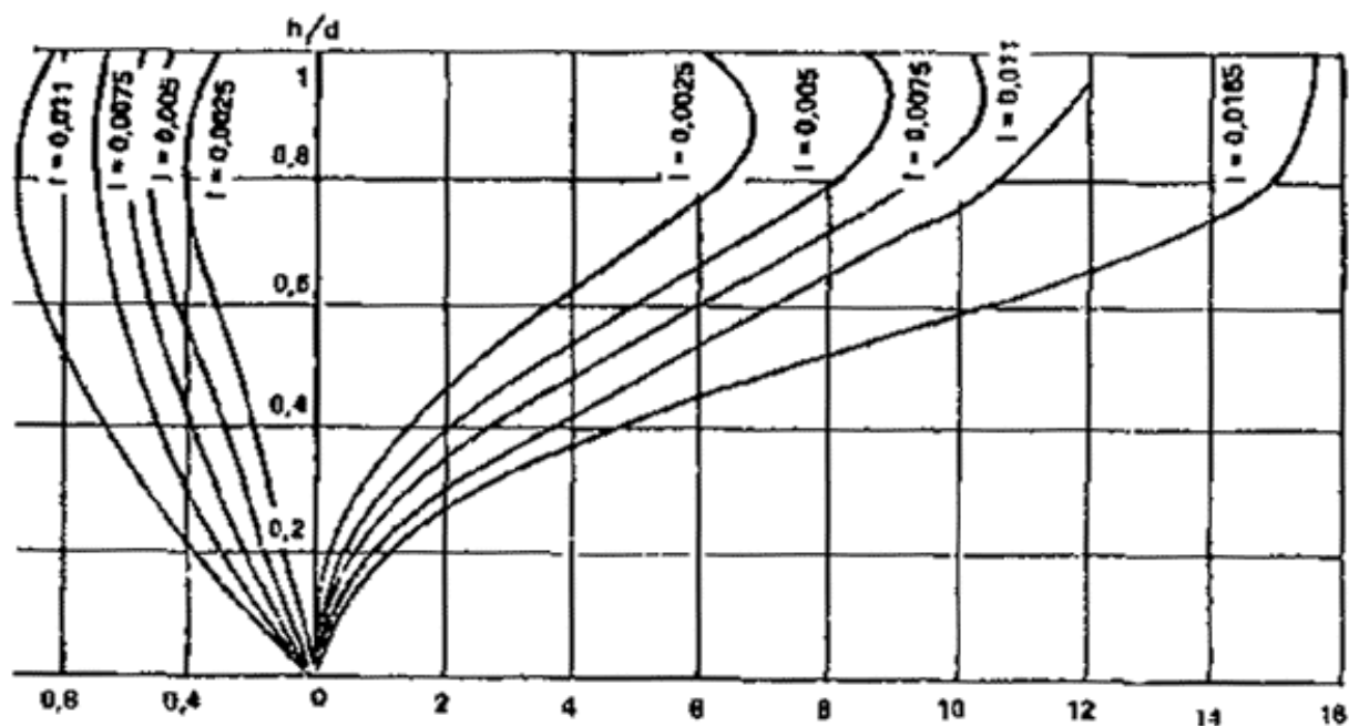
Рис. 134. График для гидравлического расчета горизонтального дренажа из трубофилтров диаметром 150 мм
