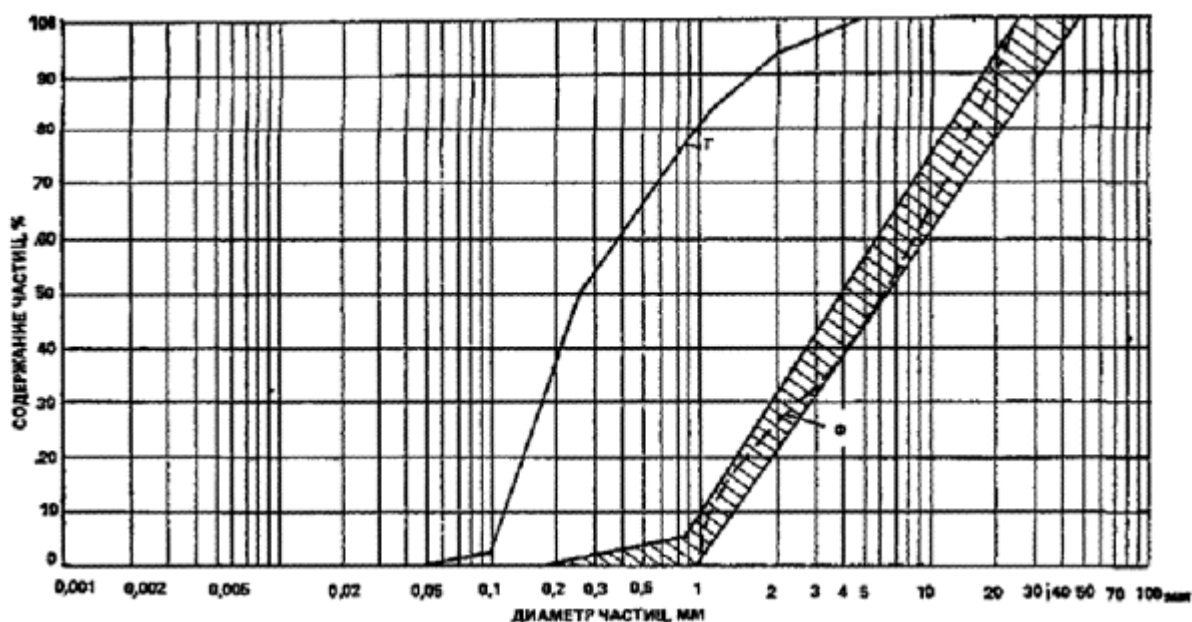
Рис. 135. Кривые гранулометрического состава к примеру подбора зернового состава фильтра для несвязанного несущего грунта
