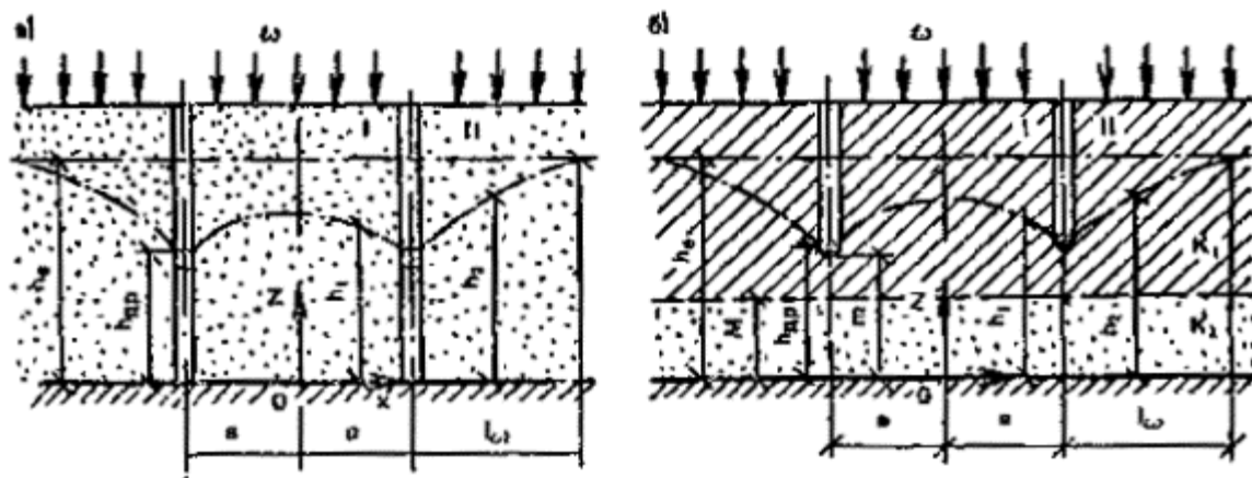
Рис. 73. Расчетные схемы двухлинейного дренажа
