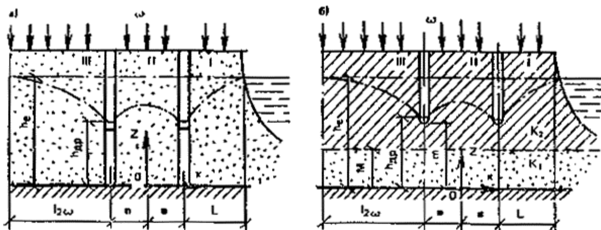
Рис. 75. Расчетные схемы двухлинейного берегового дренажа
