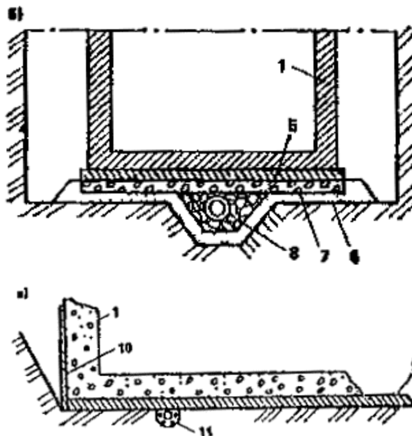
Рис. 27. Конструктивные схемы пластовых дренажей
