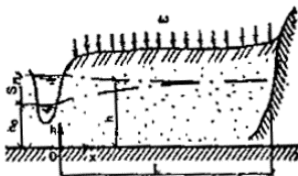
Рис. 19. Подпор грунтовых вод в долинах рек
