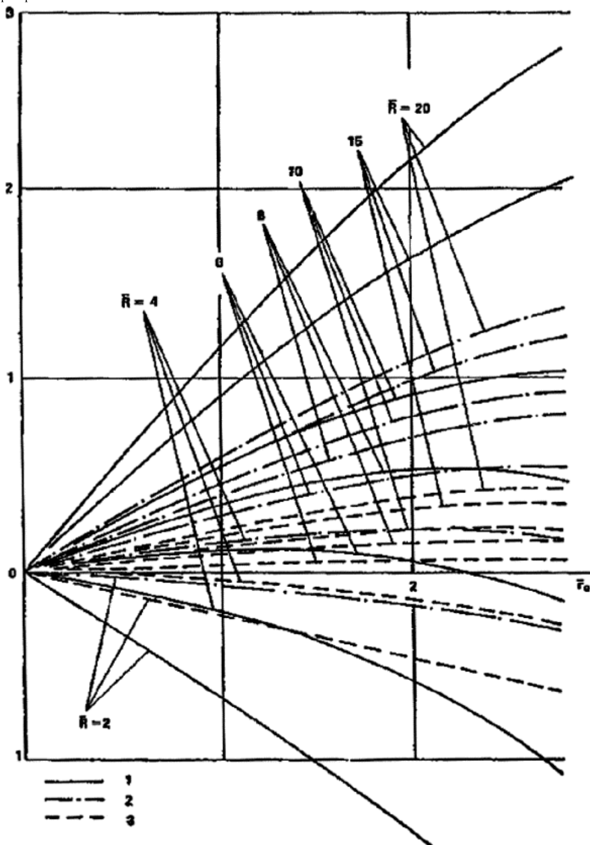
Рис. 92. График функции \Phi_{14}(\bar{R}, \bar{r}_0, \delta)
