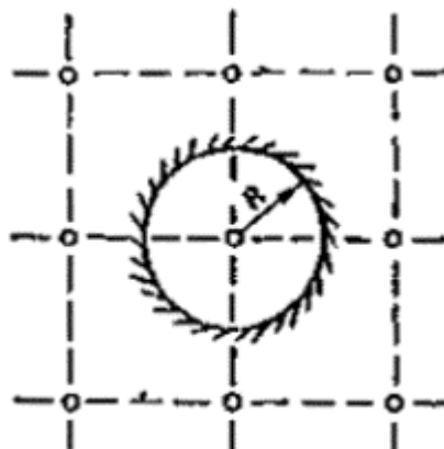
Рис. 116. Систематический вертикальный дренаж
