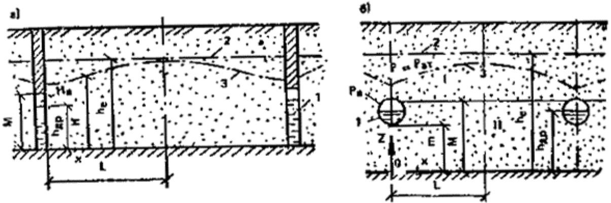
Рис. 101. Схема к расчету совершенного (а) и несовершенного (б) горизонтального вакуумного дренажа при затопленном режиме
