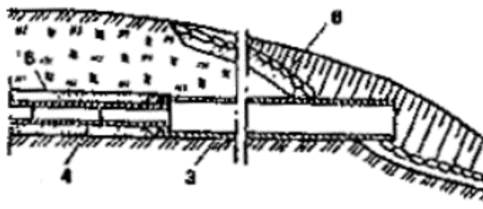
Рис. 62. Конструктивные схемы устьевых выпусков дренажных вод
