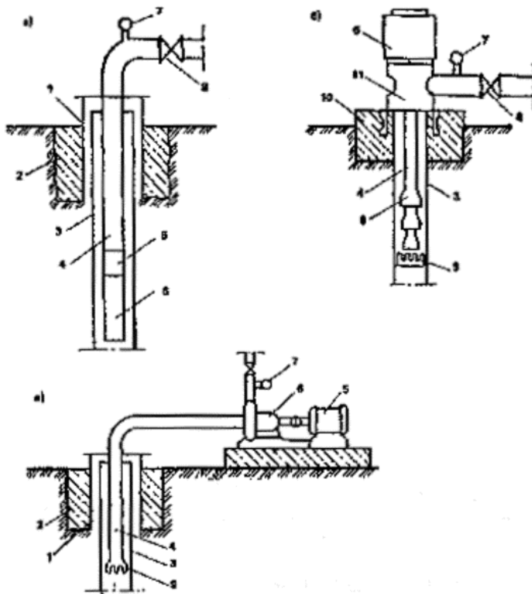
Рис. 49. Схемы оборудования дренажных скважин насосами
