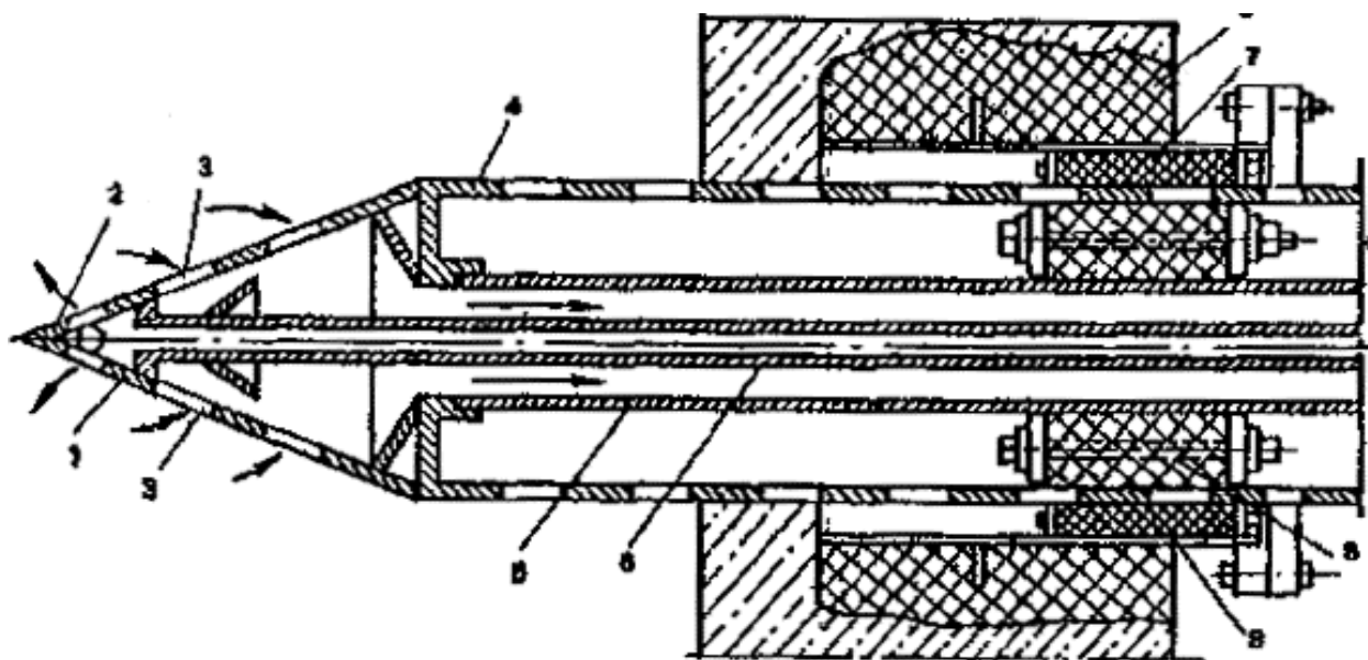
Рис. 43. Схематический разрез конуса для гидробурения лучевых дрен и детали прохода трубы в стенке колодца
