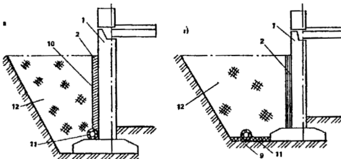
Рис. 26. Конструктивные схемы пристенных дренажей
