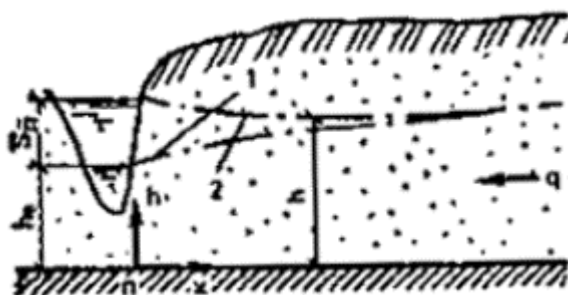
Рис. 18. Подпор грунтовых вод в полубесконечном массиве
