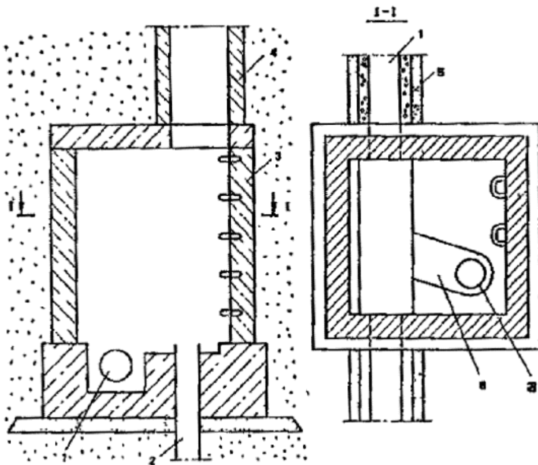
Рис. 53. Конструктивная схема комбинированного дренажа
