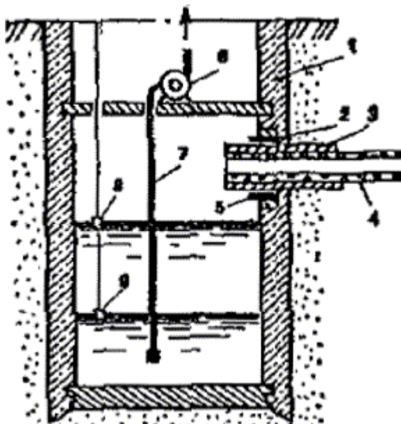
Рис. 42. Схема устройства приустьевой части лучевой дрены
