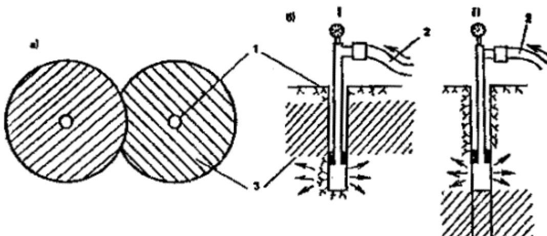
Рис. 33. Схема устройства инъекционной завесы
