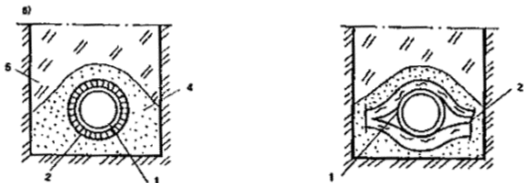
Рис. 38. Конструкции трубчатого горизонтального дренажа с фильтрующими обертками из волокнистых материалов
