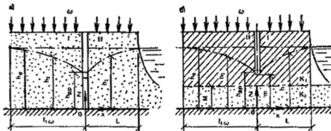
Рис. 74. Расчетные схемы однолинейного берегового дренажа
