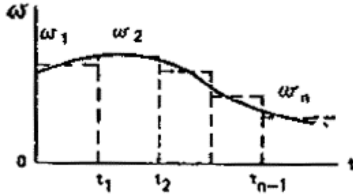
Рис. 8. Замена непрерывной функции изменения дополнительной инфильтрации ступенчатой
