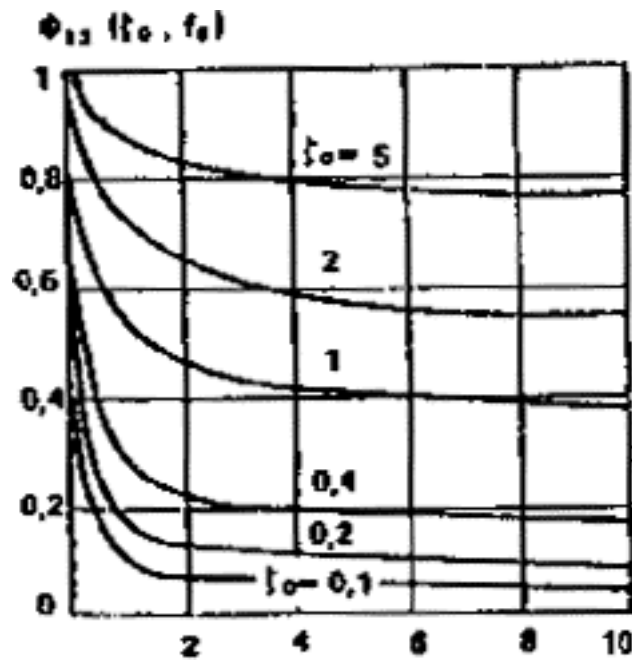
Рис. 93. График функции \Phi_{15}(\zeta_0, f_0)
