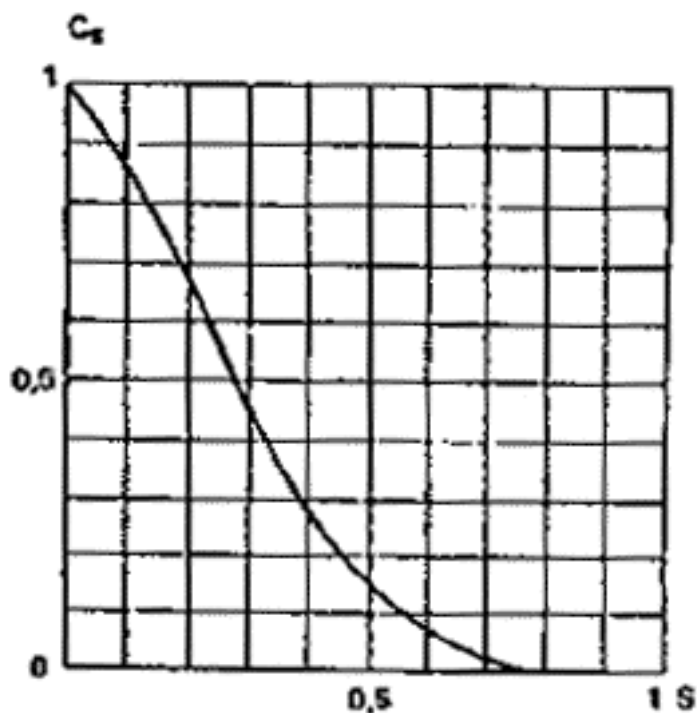
Рис. 98. График зависимости относительной проницаемости для воздуха c_s от водонасыщенности
