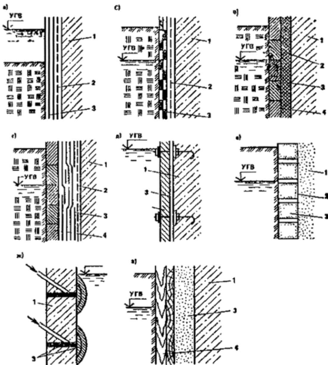
Рис. 25. Типы поверхностной гидроизоляции
