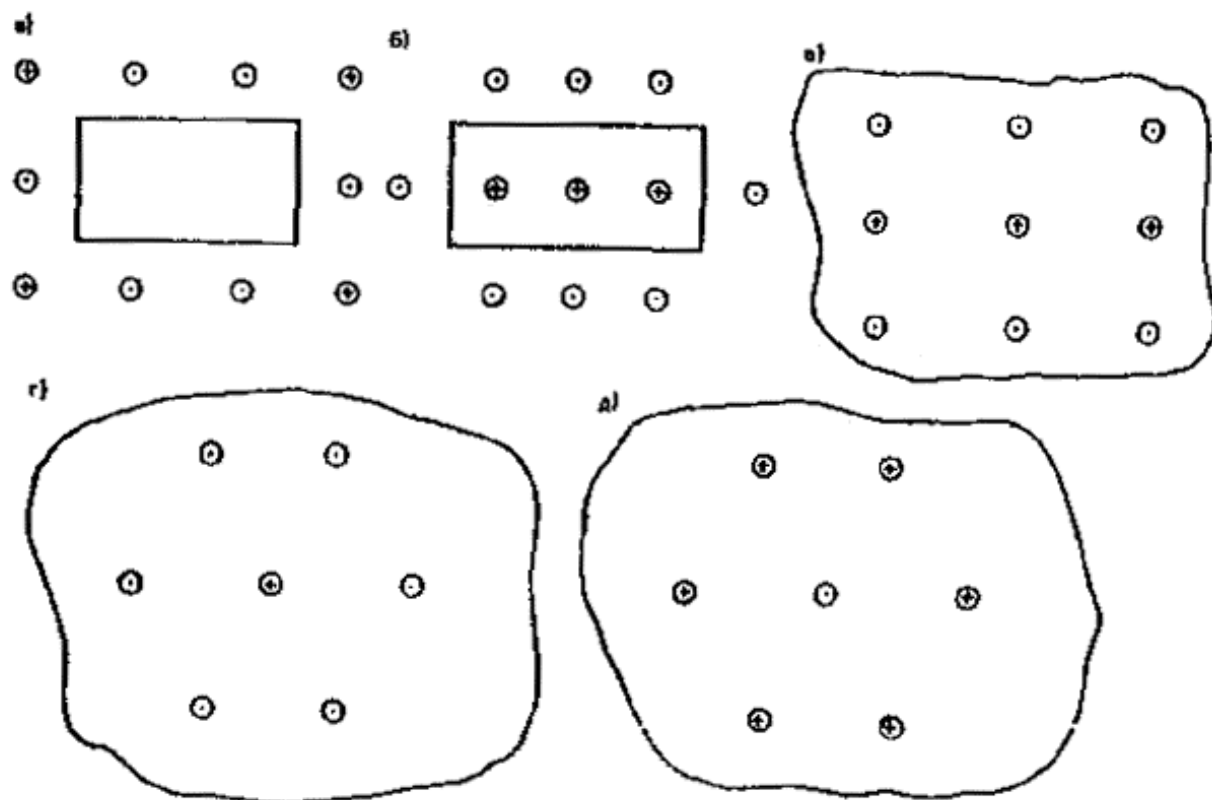
Рис. 56. Схемы планового расположения скважин пневмонагнетательных дренажей
