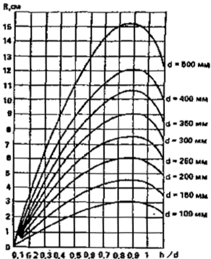
Рис. 133. График зависимости величины гидравлического радиуса R от величины относительной глубины наполнения h/d для трубофилтров различных диаметров
