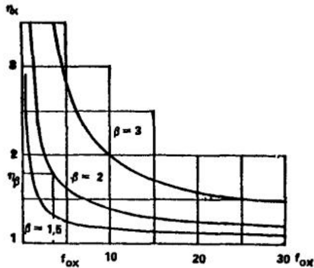
Рис. 23. График зависимости \eta_x от f_{0x}
