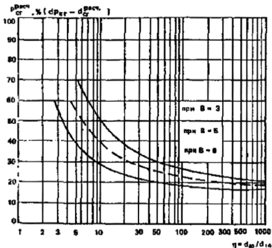
Рис. 124. График p_{гр}^{расч} = f(\eta) для определения расчетных размеров сводообразующих частиц грунта d_{гр}
