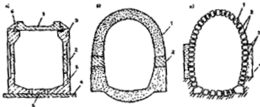
Рис. 45. Конструкция проходных дренажных галерей
