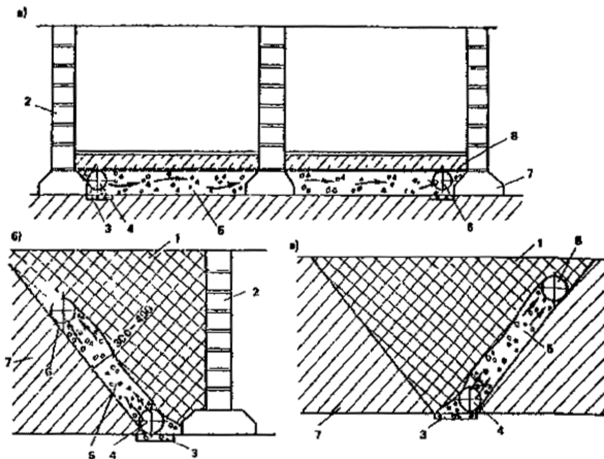
Рис. 29. Типы вентиляционного дренажа
