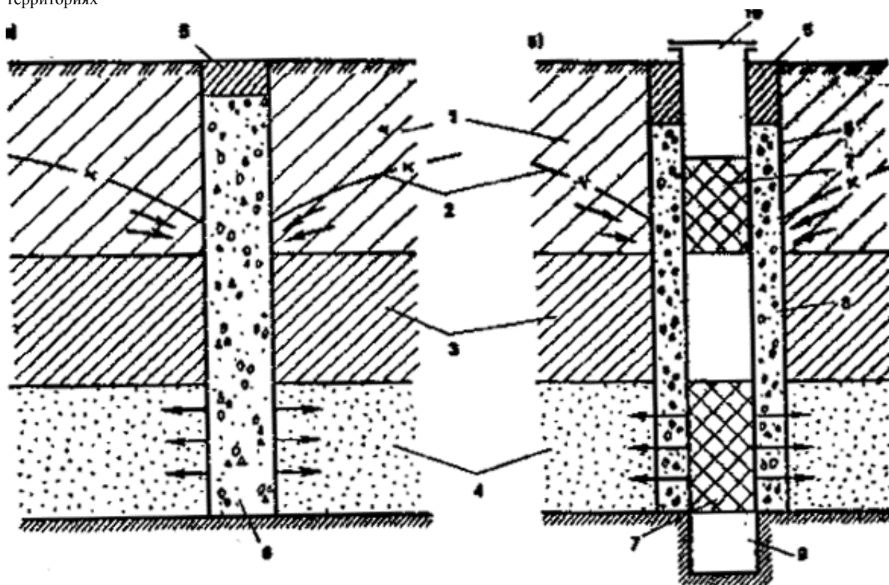
Рис. 47. Схемы конструкций вертикальных поглощающих дренажных скважин
