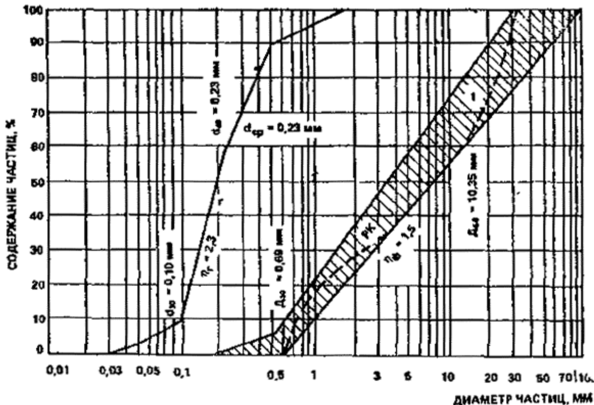
Рис. 126. График запроектированного состава фильтра
