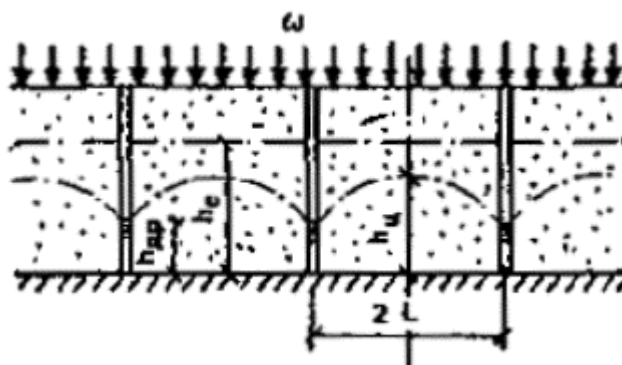
Рис. 64. Схема совершенного систематического дренажа
