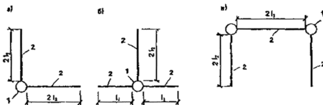
Рис. 96. Схемы (в плане) многлучевых дренажей с несимметричным расположением дрен-лучей
