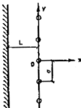
Рис. 114. Линейный ряд скважин в полуограниченном пласте
