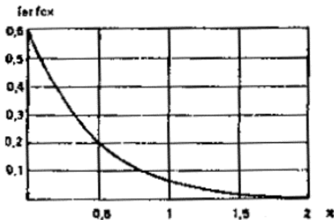
Рис. 11. График функции \text{ierfc } x .
