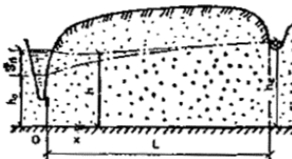
Рис. 21. Подпор грунтовых вод в междуречном массиве
