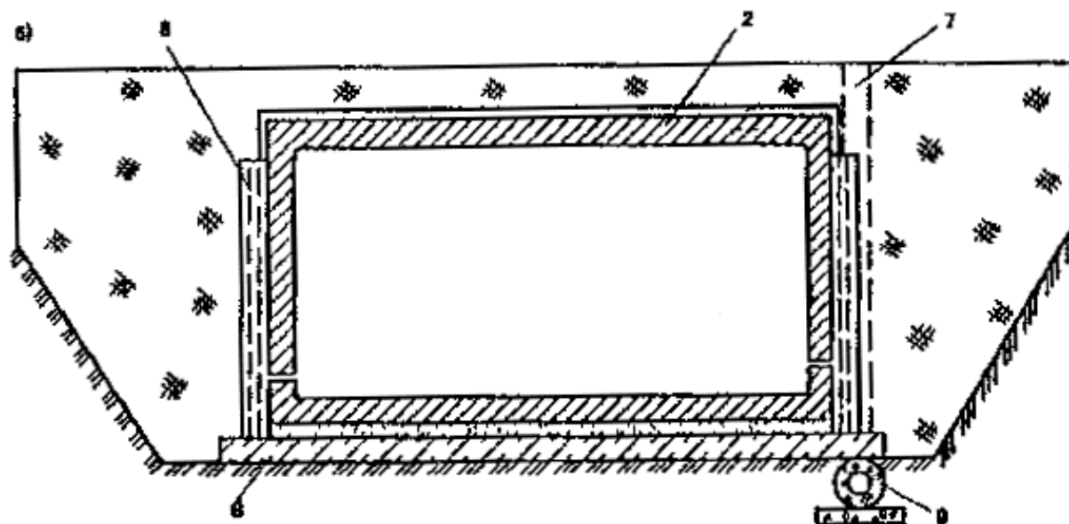
Рис. 28. Конструктивные схемы пластовых сопутствующих дренажей
