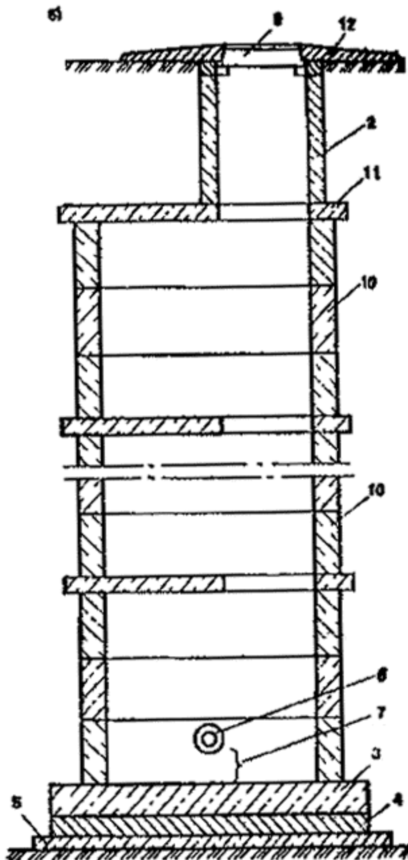
Рис. 60. Схема конструкции смотрового дренажного колодца
