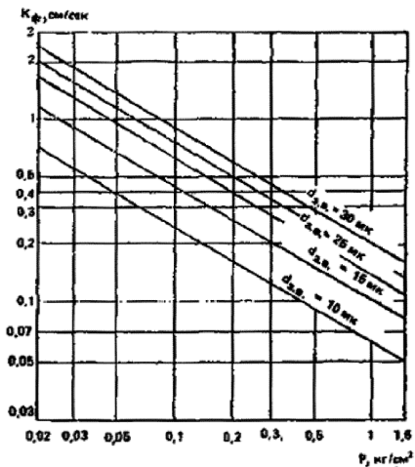
Рис. 130. График зависимости k_{\phi} = f(P, d_{э.в.})
