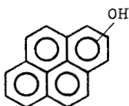
pyrenol
