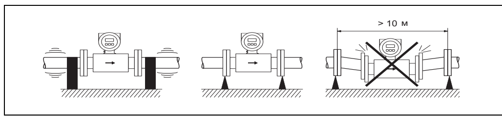
Меры для предотвращения вибрации измерительного прибора
