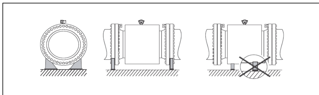
Поддержка для больших номинальных диаметров ( ДУ \geq 350 )
