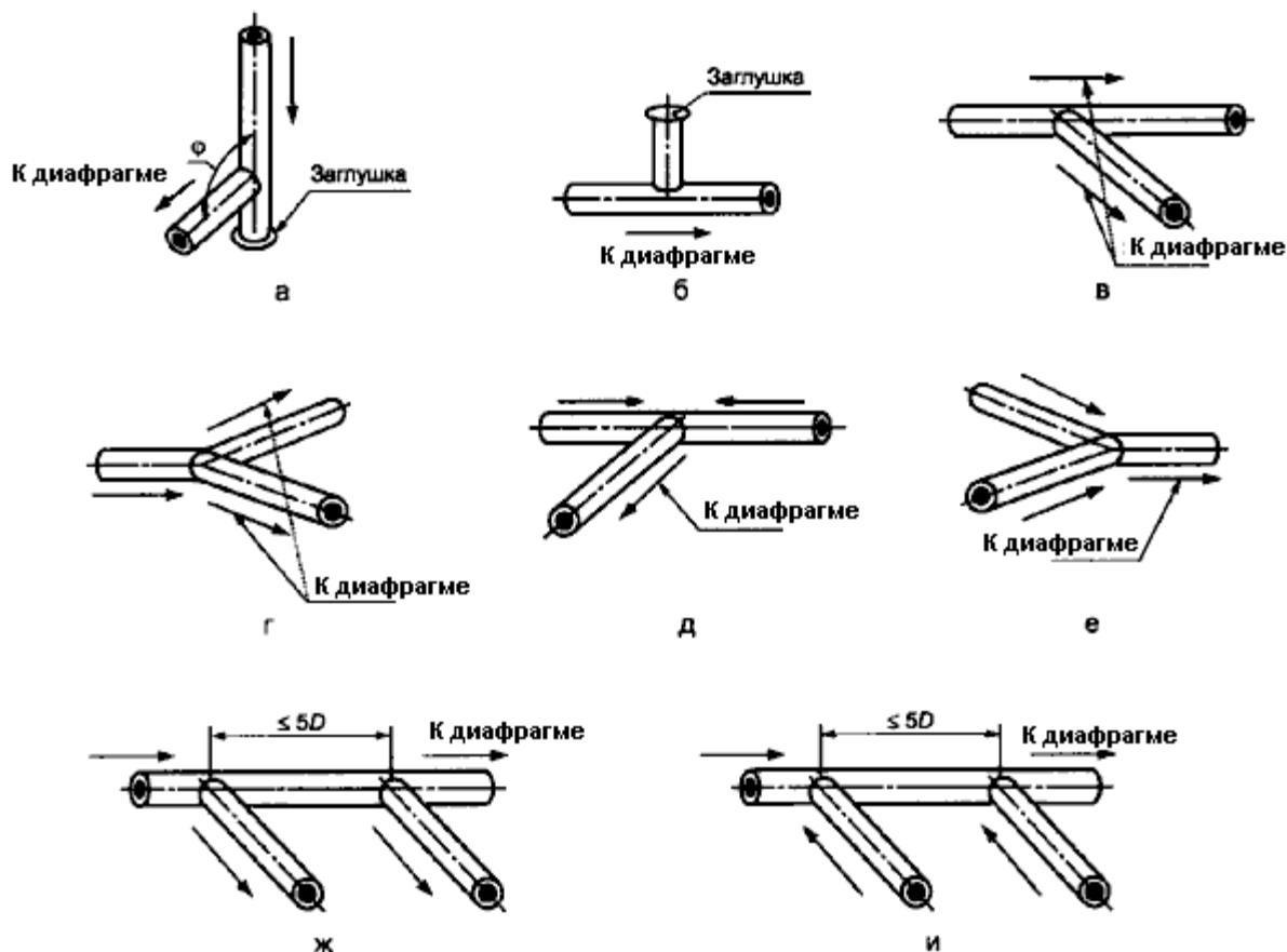
Рисунок А.2 - Тройники
