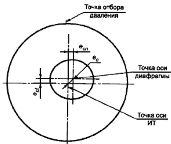
Рисунок 10 - Параметры эксцентриситета установки диафрагмы
