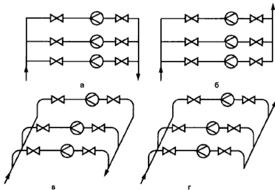
Рисунок А.4 - Схемы коллекторных систем
