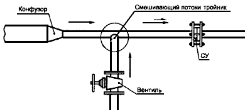
Рисунок А.7 - Возможная схема установки местного сопротивления вида "Смешивающий потоки тройник" перед сужающим устройством
