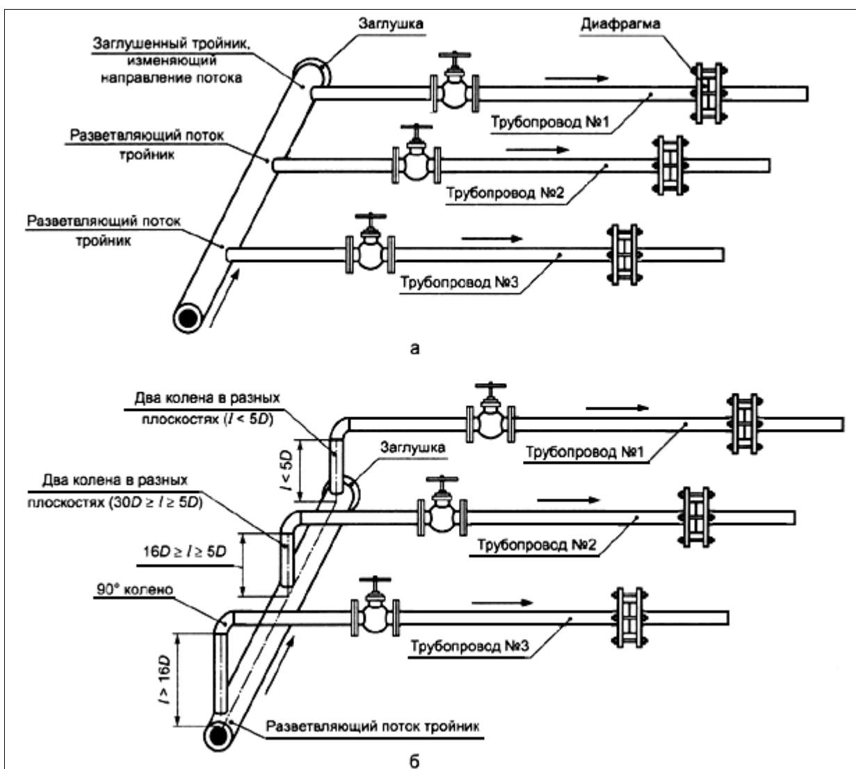
Рисунок 6 - Схема коллектора
