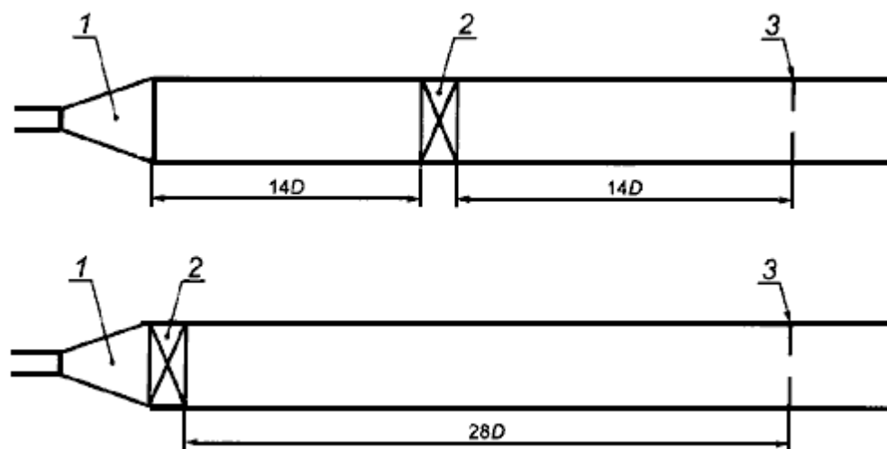
Рисунок 5 - Схема расположения шарового крана или задвижки при \beta = 0,6
