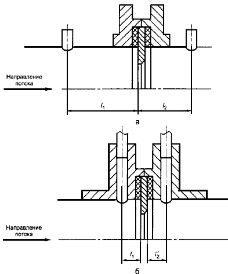
а - трехрадиусный отбор; б - фланцевый отбор
