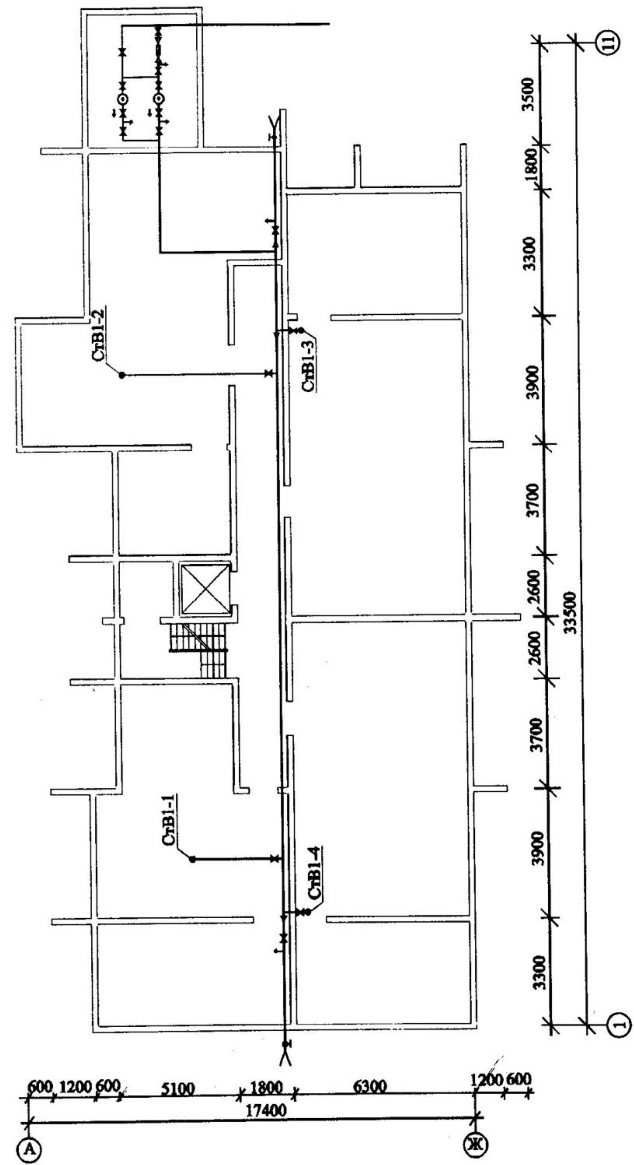
Рис. 6. План подвала
