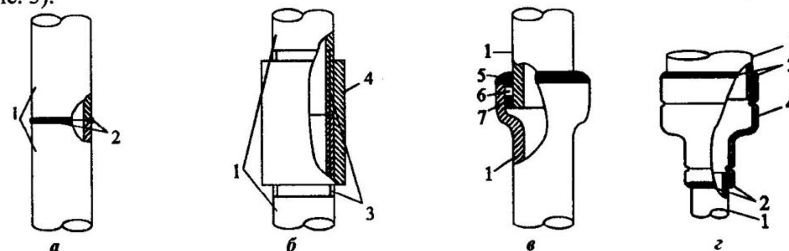
Рис. 3. Виды соединений водопроводных труб: а – на сварке; б – резьбовое; в – раструбное; г – переходная муфта; 1 – труба, 2 – сварной шов, 3 – резьба, 4 – муфта, 5 – асестоцементная смесь, 6 – белая прядь, 7 – просмоленная прядь
