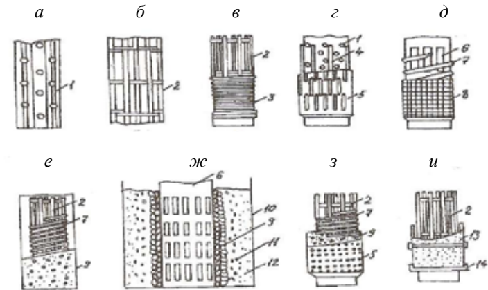
Рис. 11. Некоторые типы фильтров трубчатых колодцев: а – трубчатый фильтр с круглой перфорацией; б – каркасно-стержневой фильтр; в – проволочный фильтр со стержневым каркасом; г – фильтр из стального штампованного листа с трубчатым каркасом; д – сетчатый фильтр с трубчатым каркасом со щелевой перфорацией и проволочной обмоткой; е – однослойный гравийный фильтр со стержневым каркасом и проволочной обмоткой; ж – многослойный гравийный фильтр с трубчатым каркасом со щелевой перфорацией; з – кожуховый гравийный фильтр со стержневым каркасом, проволочной обмоткой, однослойной гравийной обсыпкой и водоприемной поверхностью из стального штампованного листа; и – блочный фильтр со стержневым каркасом; 1 – каркас трубчатый с круглой перфорацией; 2 – стержневой каркас; 3 – проволочная обмотка; 4 – подкладочные продольные стержни; 5 – стальной штампованный лист с продольными отверстиями; 6 – трубчатый каркас со щелевой перфорацией; 7 – подкладочная проволочная обмотка; 8 – сетка; 9 – гравийная обсыпка; 10 – обсадная труба; 11 – крупнозернистый песок; 12 – песок среднезернистый; 13 – блоки из пористого бетона; 14 – резиновые уплотнительные прокладки
