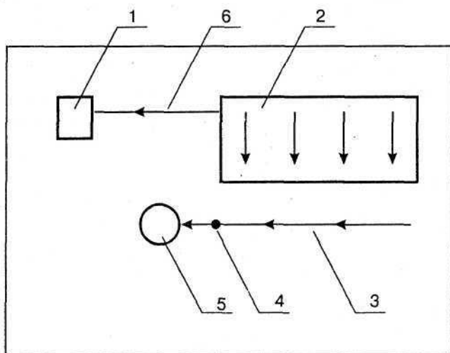
Рис. 10. Схема отвода атмосферных осадков: 1 — земельный участок; 2 — кровля здания; 3 — самотечная канализация отвода атмосферных осадков; 4 — спусковой стояк; 5 — резервуар для атмосферных осадков; 6 — самотечная канализация хозяйственно-бытовых стоков
