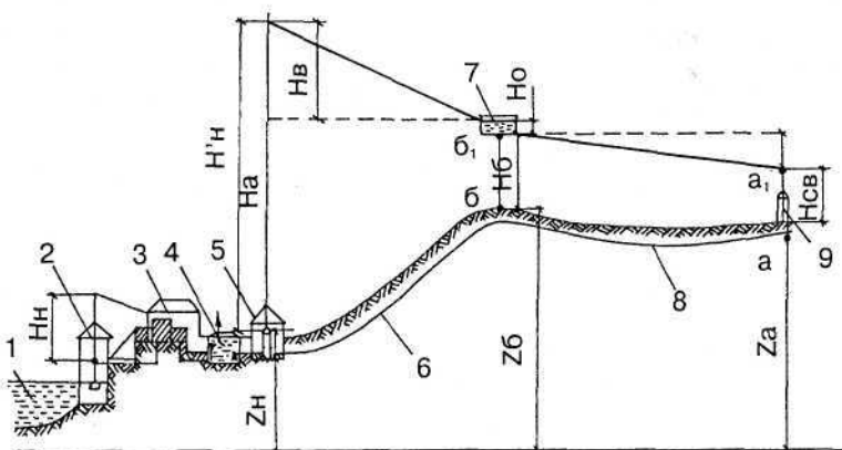
Рис. 3. Положение геометрических линий при максимальном водоразборе: 1 — источник водоснабжения; 2 — водоприемник, совмещенный с насосной станцией 1-го подъема; 3 — водоочистные сооружения; 4 — резервуар чистой воды; 5 — насосная станция 2-го подъема; 6 — напорный водовод; 7 — водонапорная башня; 8 — распределительная сеть; 9 — объекты водопотребления; H_{св} — свободный напор излива у водозаборного прибора потребителя (метры водяного столба); H_b — расчетная высота водонапорной башни (метры водяного столба); H_a — высота столба воды в водонапорной башне (метры водяного столба); H_v — потери напора в водопроводе (метры водяного столба); H_n — требуемый напор подачи воды насосом (метры водяного столба); Z_n , Z_b , Z_a — высота подъема воды от горизонта забора до поверхности земли
